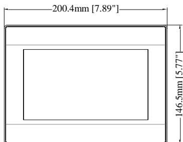
正视图
