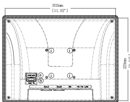
背视图
