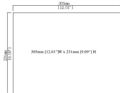
开孔尺寸图
