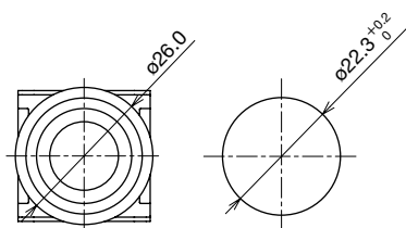
安装孔加工图
