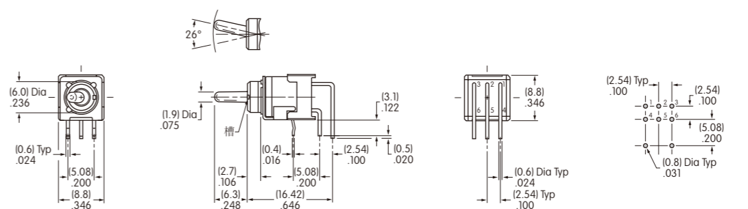
直角型PC端子
