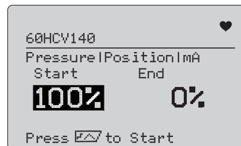
图示 56. 扰动 / 局部试验
