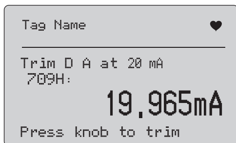
图示 40. 20 mA 微调屏幕
