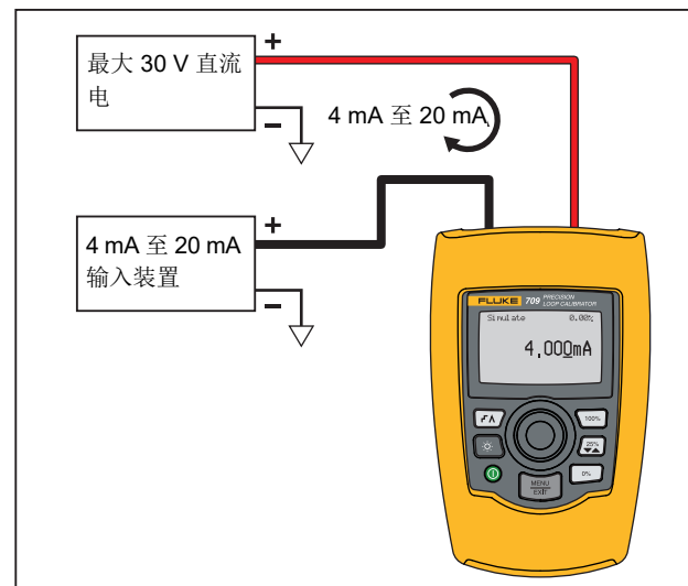
图示 5. mA 模拟连接
