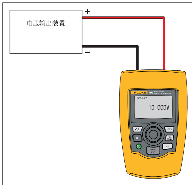
图示 8. 电压测量连接
