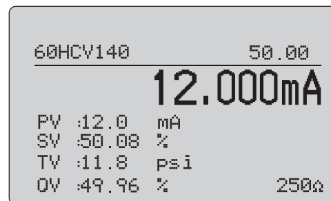
图示 53. 手动测试
