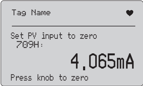
图示 42. PV 归零屏幕
