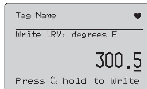
图示 33. 写入 LRV 屏幕
