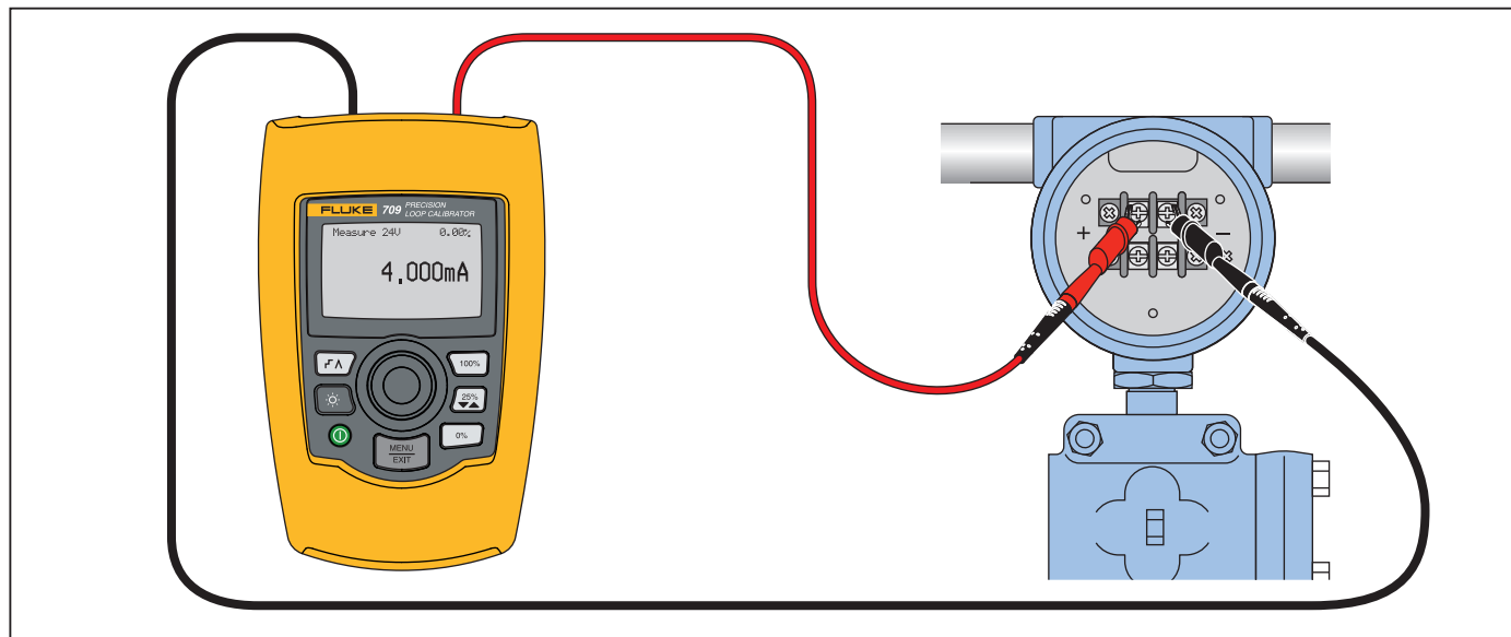
图示 7. 24 V 电压下 mA 测量连接
