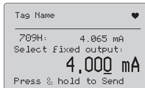
图示 41. 设置固定 mA 输出屏幕
