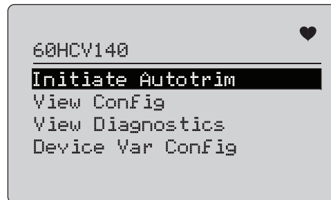
图示 58. HART 通信菜单
