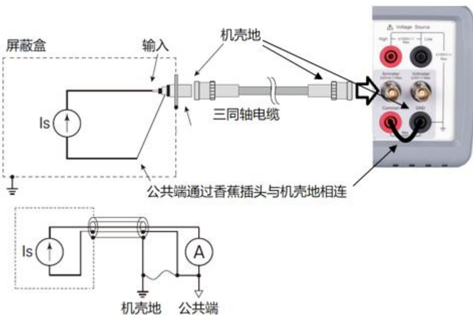
图 4-3 浮地的电流测量连接方式
