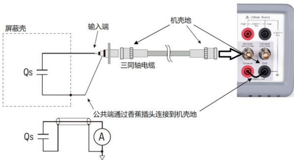
图 4-12 电荷测量的连接方式
