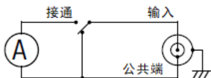
图 4-2 典型的接地的电流测量连接方式
