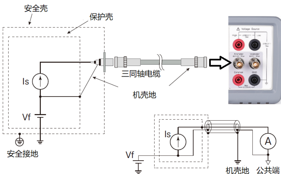
图 4-3 浮地的电流测量连接方式
