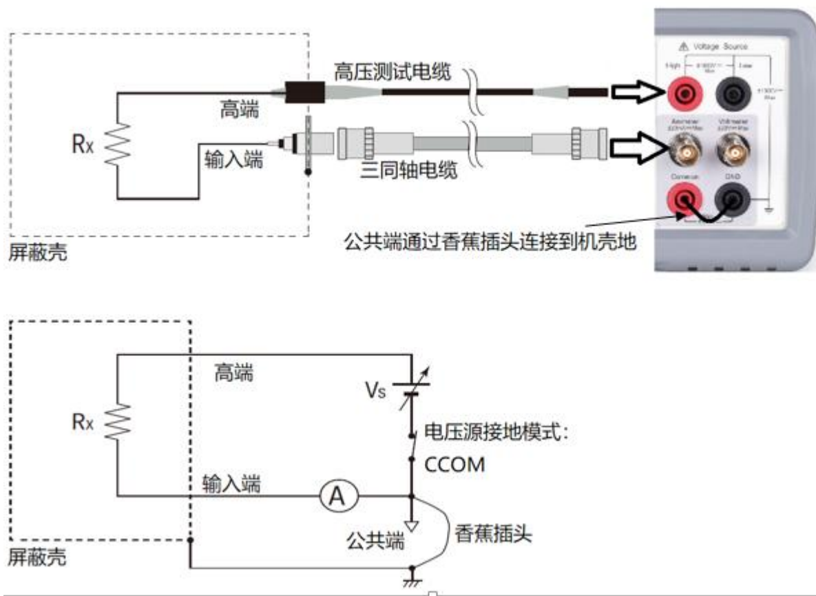
图 4-10 浮动设备的测量
