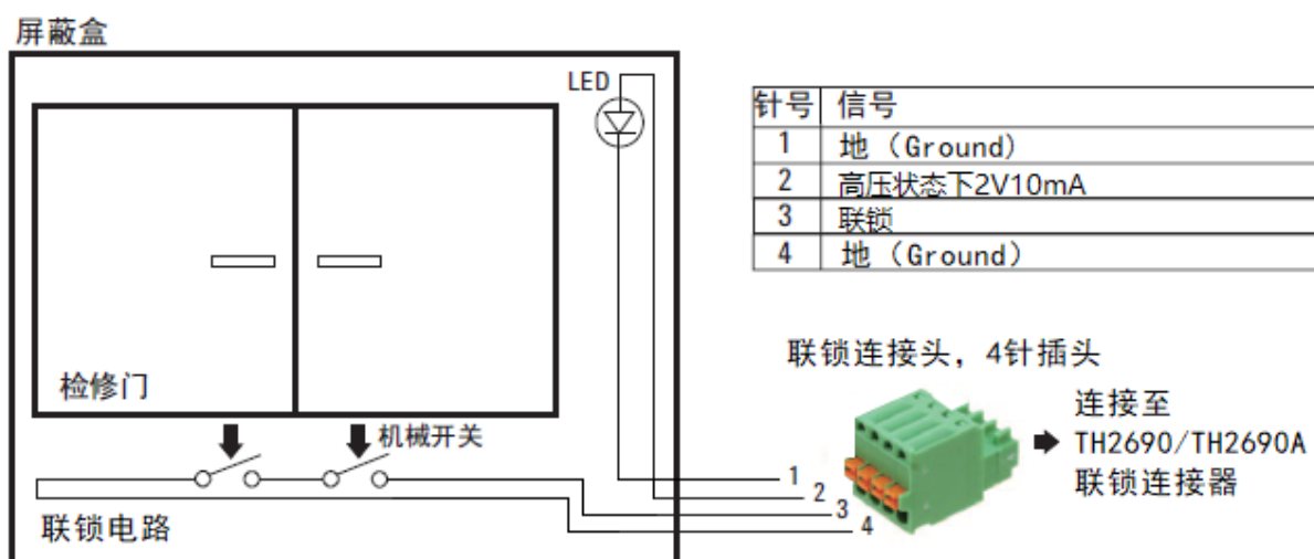
图 4-14 联锁电路
