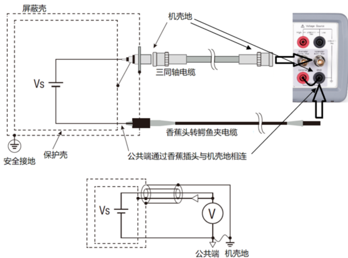
图 4-7 无保护的电压测量连接方式
