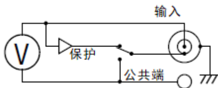
图 4-5 电压表简化电路图
