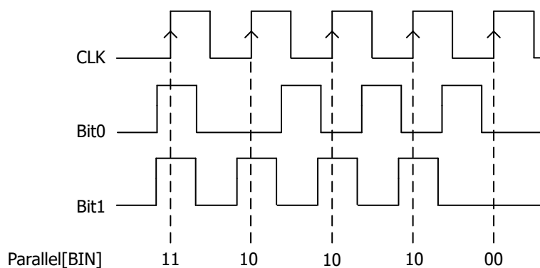
图 3.1 并行解码示意图
