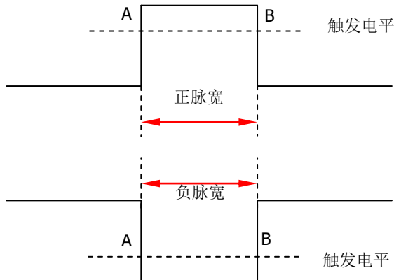
图 5-3 正脉宽/负脉宽
