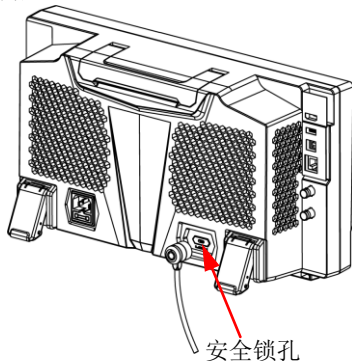
图 1-21 使用安全锁
