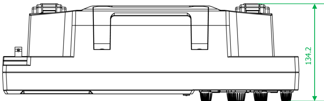
图 1-2 俯视图
