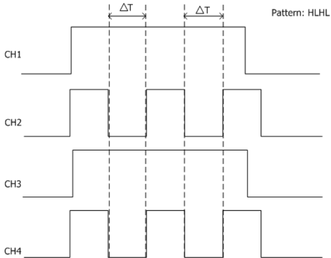
图 5-7 持续时间触发示意图
