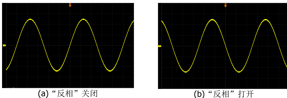
图 2-1 波形反相
