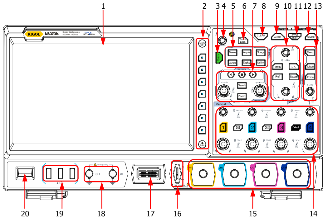
图 1-13 前面板总览
