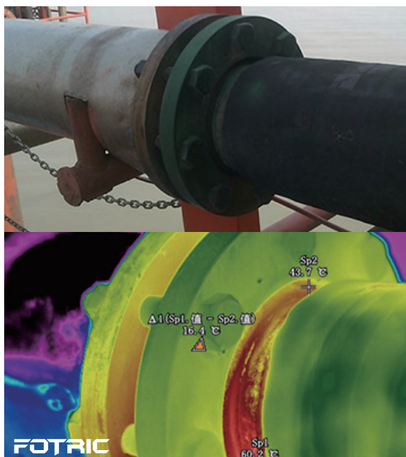
管道法兰连接处老化
