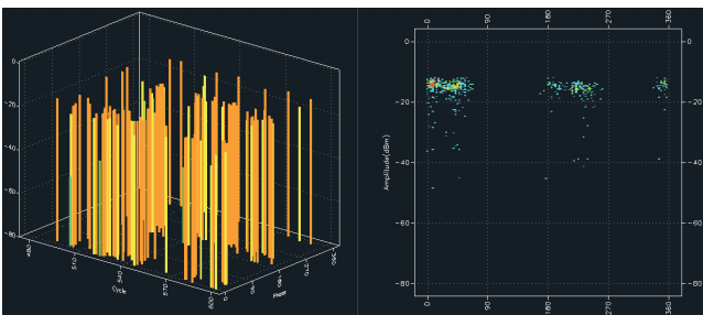
悬浮放电
