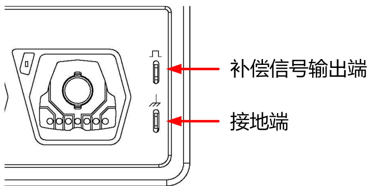
图 5.5 补偿信号
