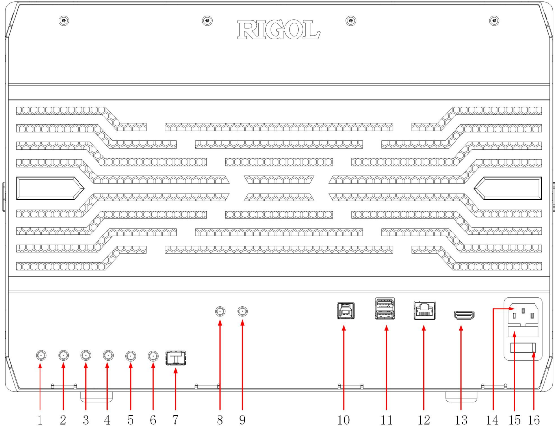
图 4.2 后面板
