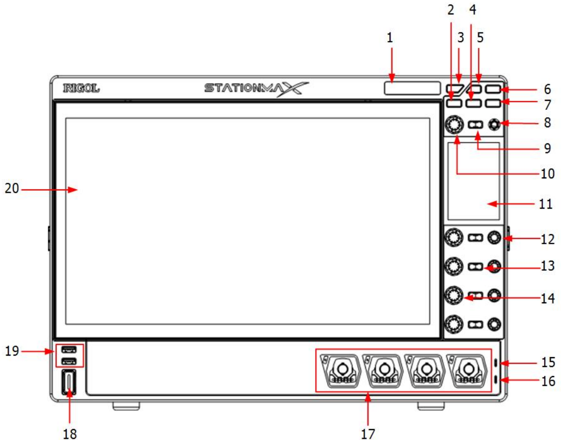
图 4.1 前面板
