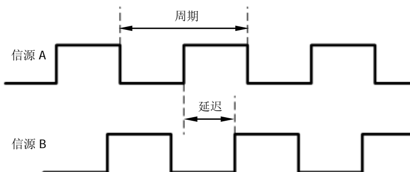
图 6-4 延迟和相位
