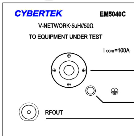
前面板
