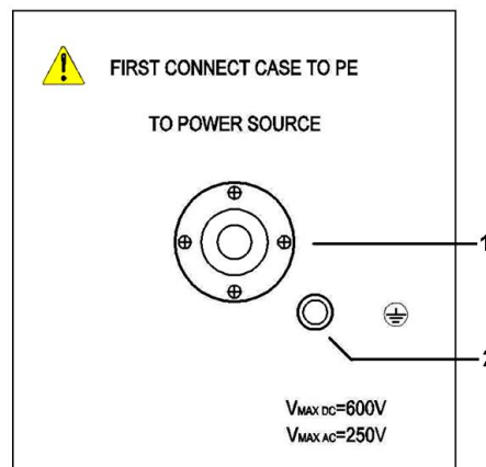
后面板
