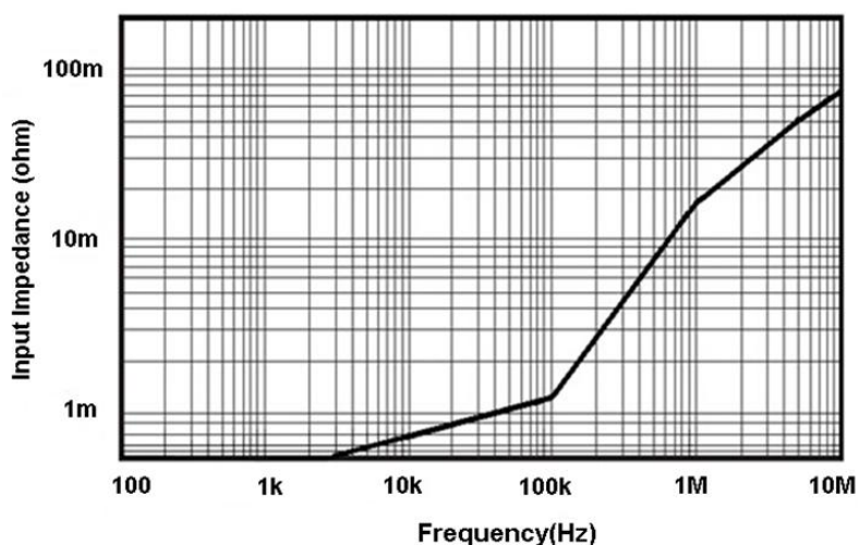
图 12 CP8500A 输入阻抗 VS 频率曲线
