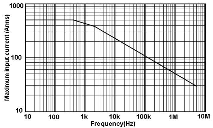
图 11 CP8500A 最大峰值电流 VS 频率曲线
