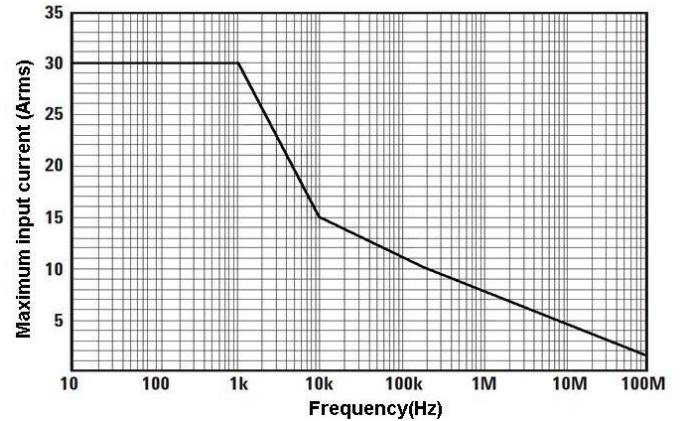
图 2.b CP8030H 最大测量电流 VS 频率曲线
