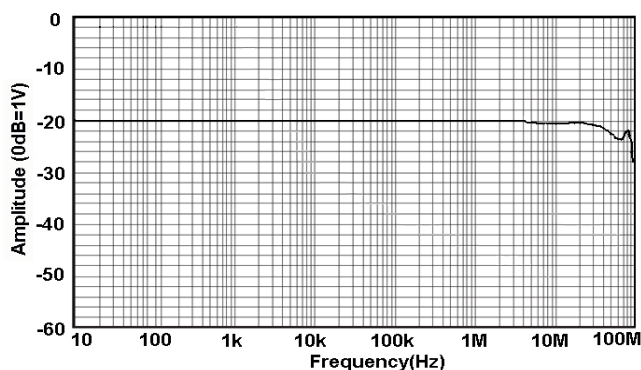
图 1.a CP8030B 幅频曲线
