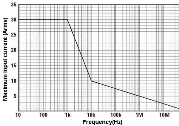
图 2.a CP8030B 最大测量电流 VS 频率曲线
