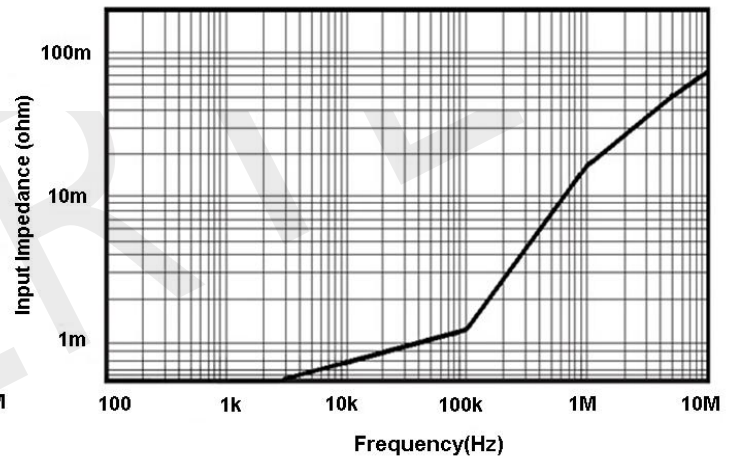
图 9 CP8300A 输入阻抗 VS 频率曲线
