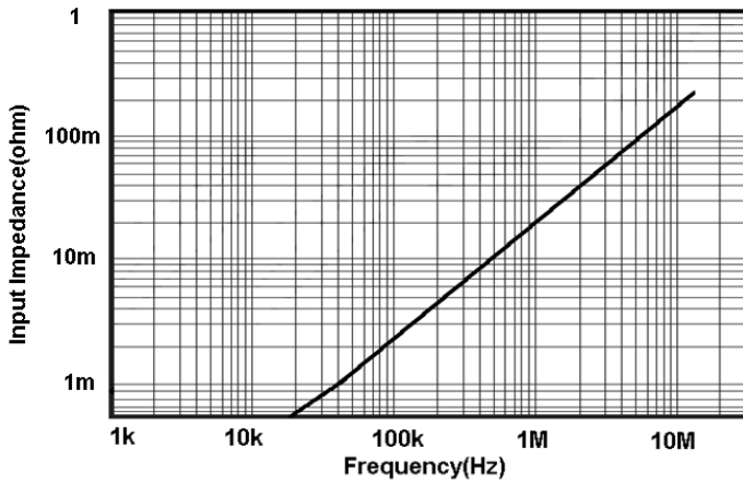
图 6 CP8150A 输入阻抗 VS 频率曲线
