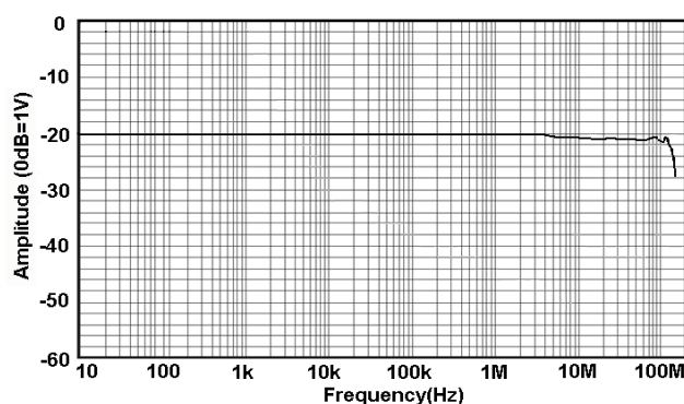
图 1.b CP8030H 幅频曲线
