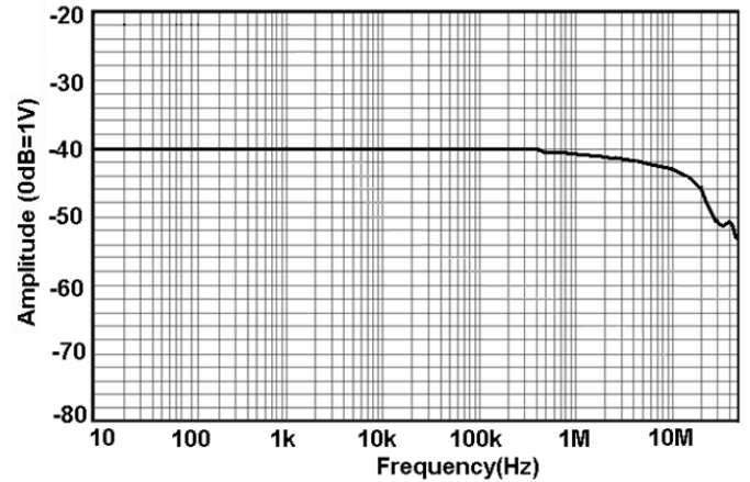
图 7 CP8300A 幅频曲线
