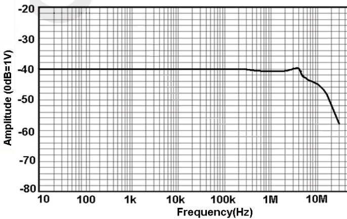
图 10 CP8500A 幅频曲线
