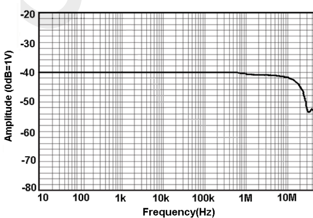
图 4 CP8150A 幅频曲线
