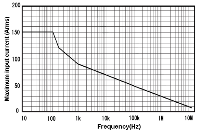
图 5 CP8150A 最大测量电流 VS 频率曲线
