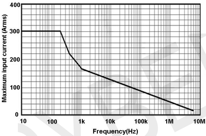
图 8 CP8300A 最大测量电流 VS 频率曲线
