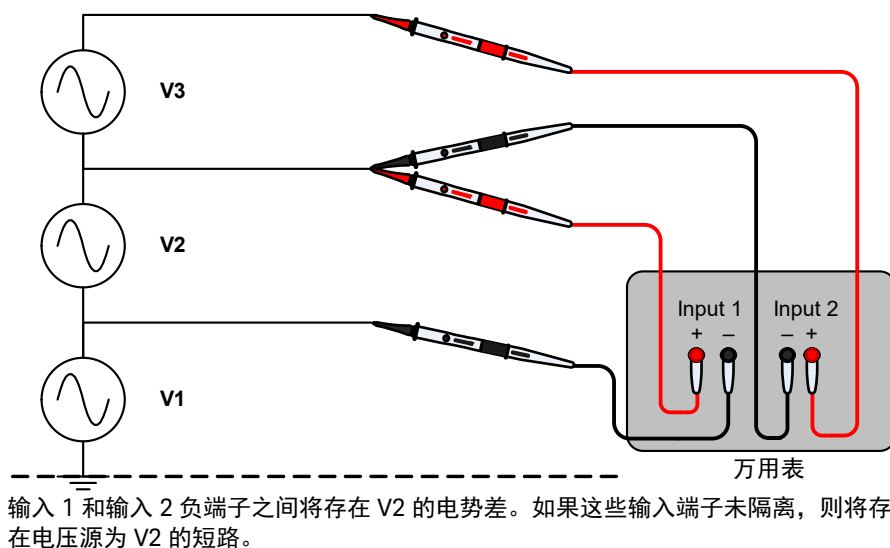
图 1-6 接地环路
