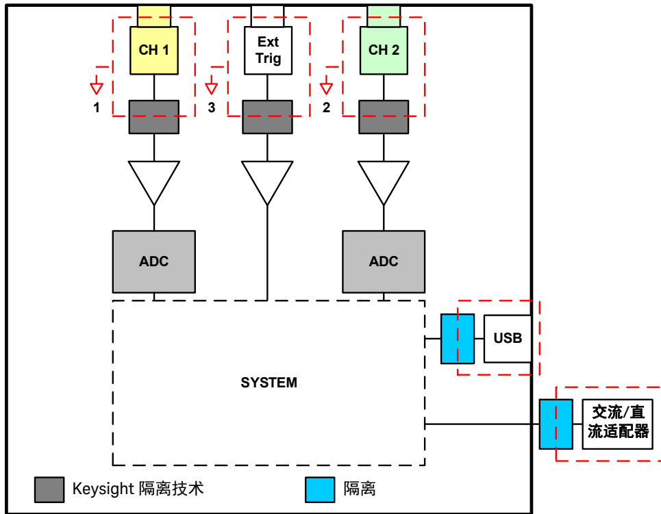
图 1-7 通道隔离块示意图
