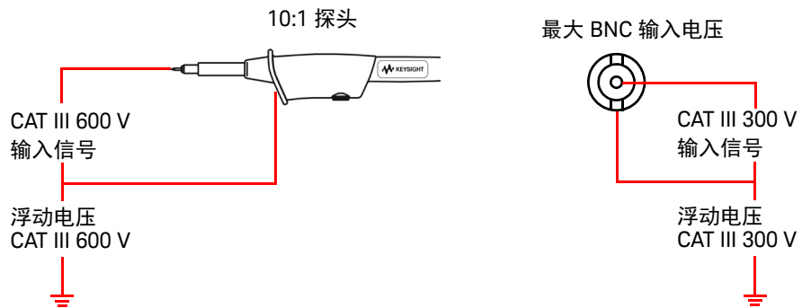
图 1-10 在 CAT III 300 V 条件下的通道到通道隔离
