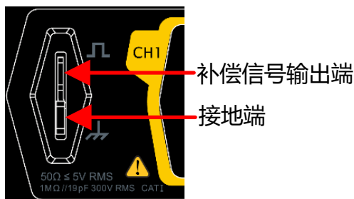
图 7.7 使用补偿信号
