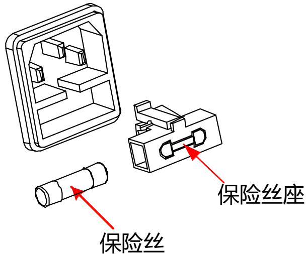
图 11.1 更换保险丝
