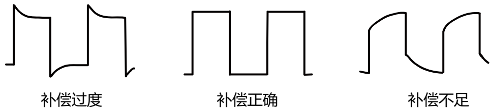
图 7.9 探头补偿
