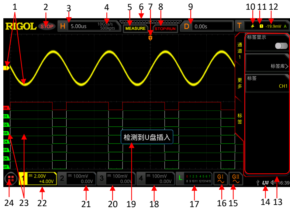
图 6.3 用户界面
