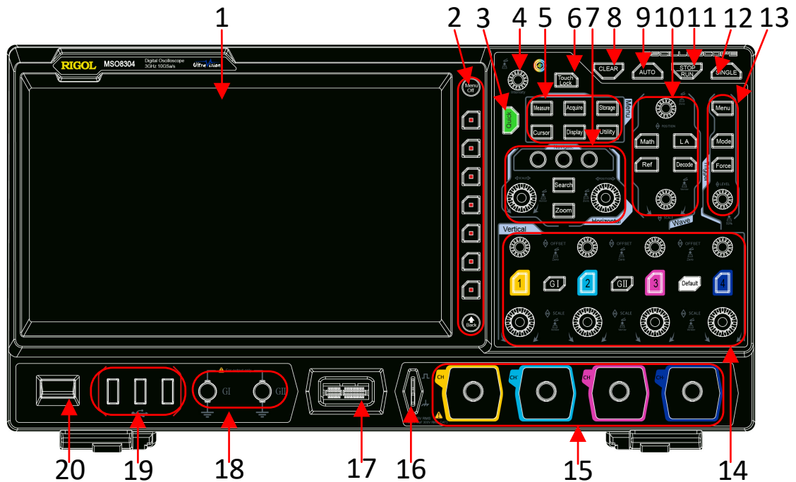
图 6.1 前面板
