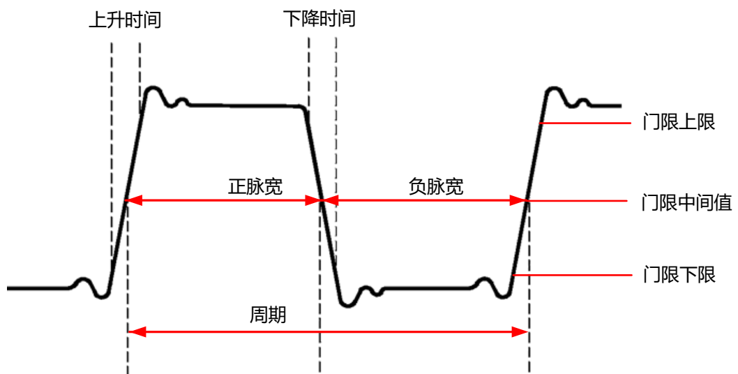
图 9.1 时间参数
