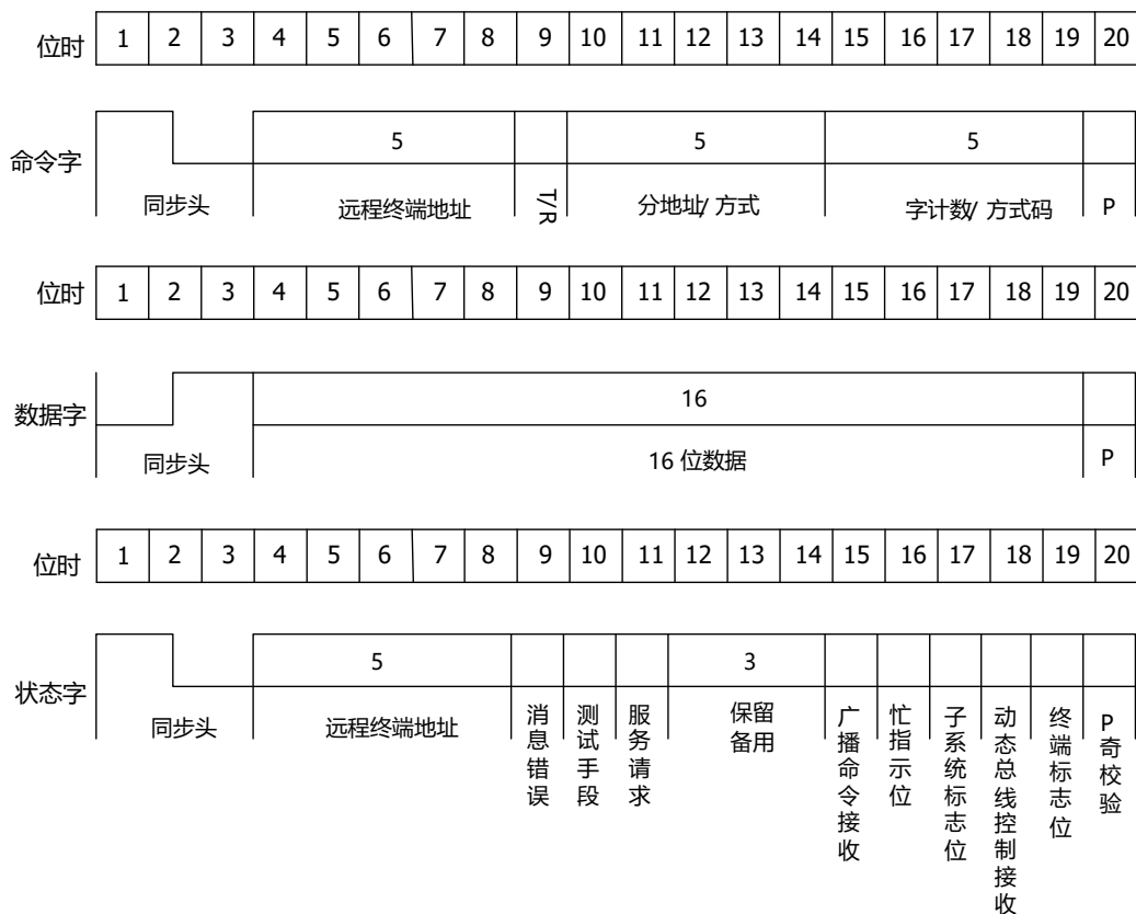
图 8.24 1553B 总线命令字、数据字和状态字格式图
