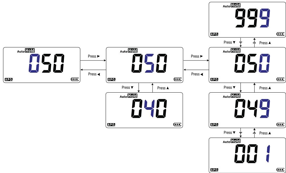
图 4-1 更改可变计数
