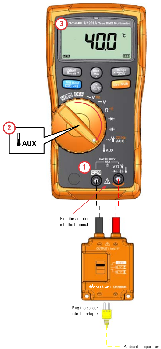
图 2-20 使用辅助温度测量功能（仅适用于 U1231A 和 U1232A 型号）
