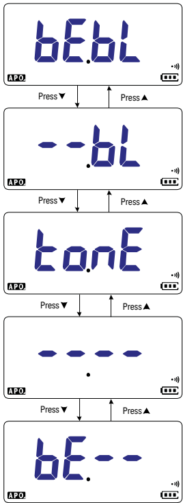
图 4-11 更改导通测试警报
