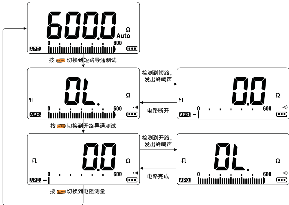
图 2-10 导通测试流程
