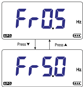
图 4-10 更改可测量的最低频率
