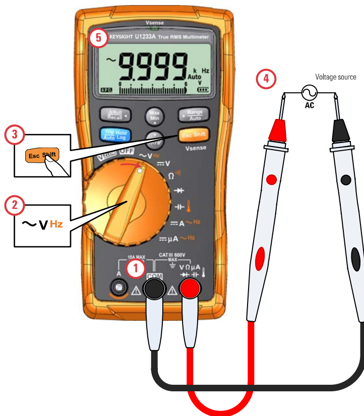
图 2-28 测量频率
