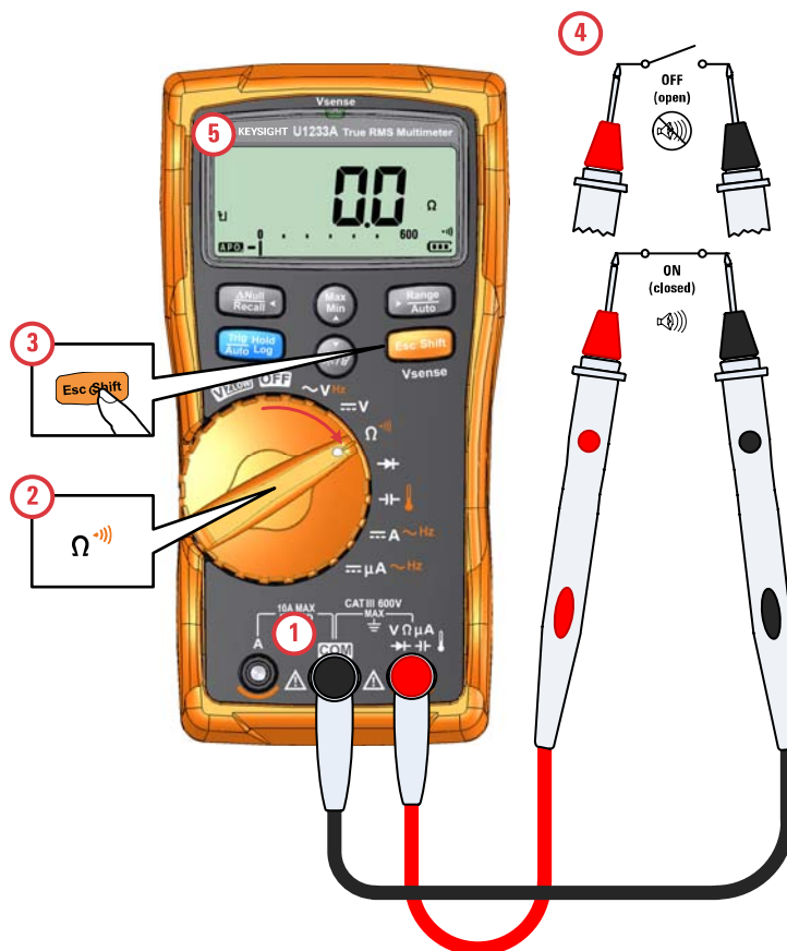
图 2-11 导通测试
