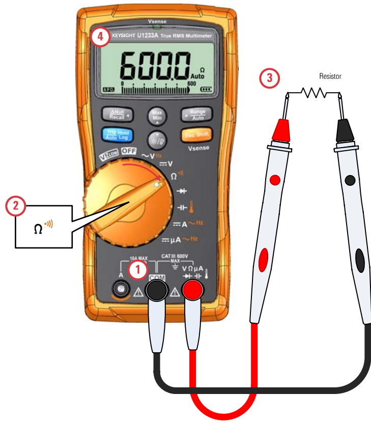
图 2-9 测量电阻
