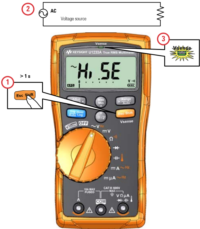
图 3-1 检测是否存在电压
