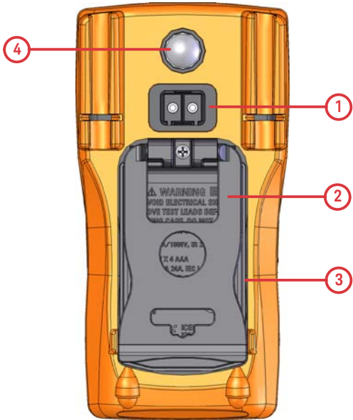
图 1-8 后面板
