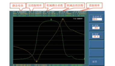
频响分析（换能器找谐振点）
