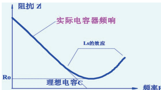
图F-2 电容器的阻抗频率
