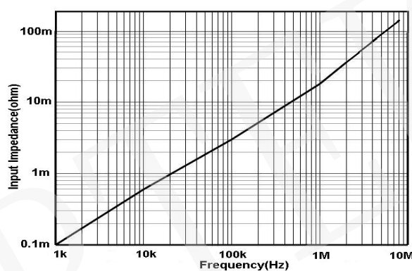
图 15.b HCPX8300A 输入阻抗 VS 频率曲线
