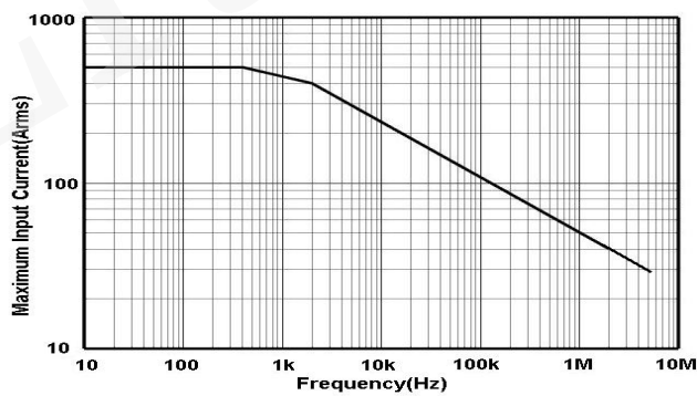
图 17 HCPX8500 最大测量电流 VS 频率曲线 (超过该曲线所示最大电流连续使用会导致探头烧毁)
