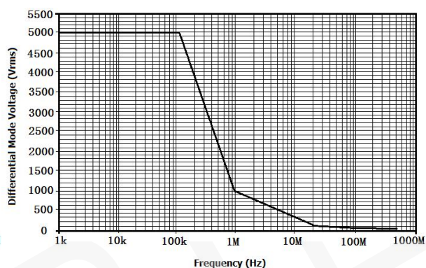
图 4 DPX6700A 最大差模电压 VS 频率
