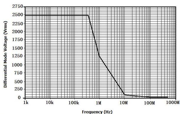
图 3 DPX6350A 最大差模电压 VS 频率
