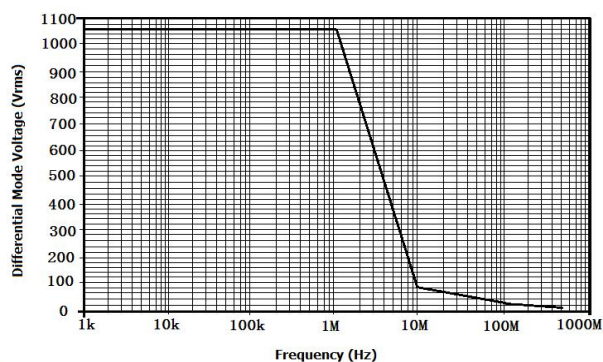
图 2 DPX6150A 最大差模电压 VS 频率
