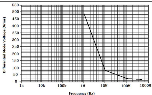
图 1 DPX6070A 最大差模电压 VS 频率
