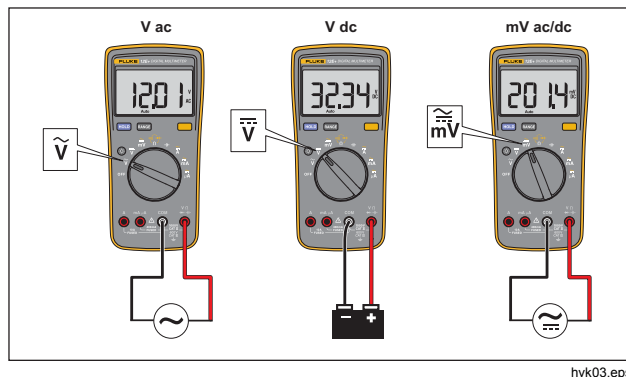
图 1. 测量交流和直流电压
