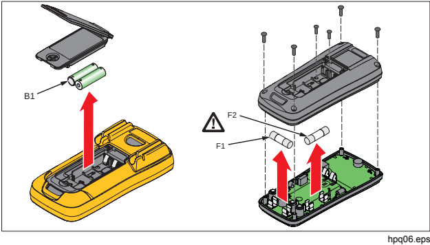
图 4. 更换电池和保险丝
