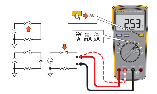
图 2. 测量交流和直流电流
