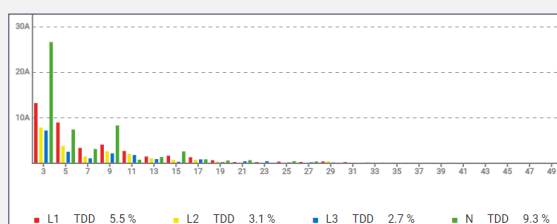
每个电流模块的所有 4 个电流的谐波/间谐波分析，也可作为 10 分钟平均值提供
