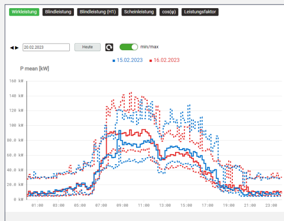
负载曲线的波动范围
