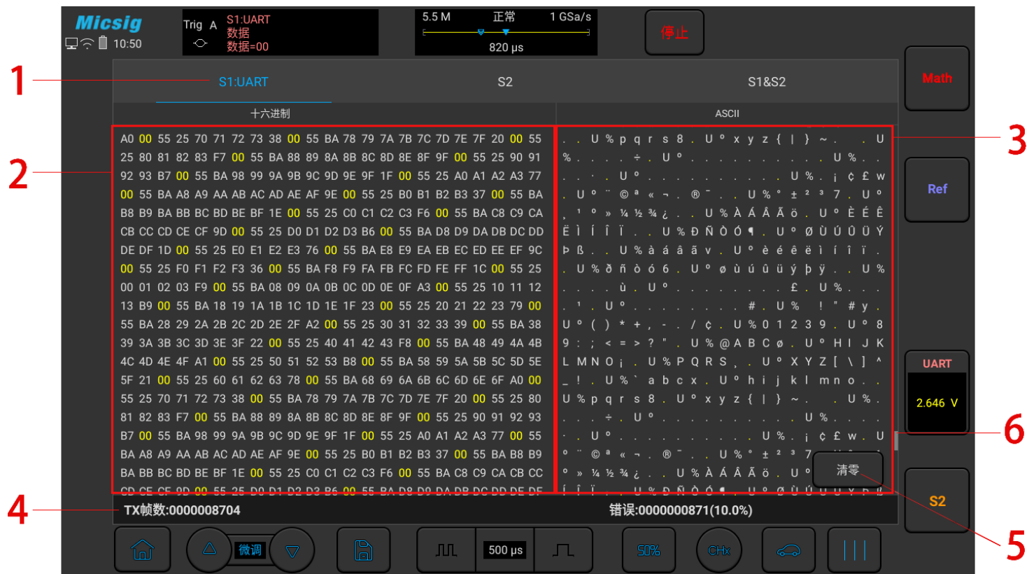
图12-9 UART 文本界面
