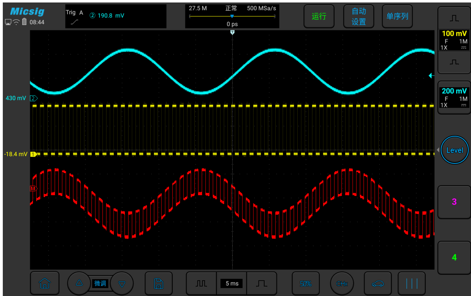
图9-2 通道 1 加通道 2 数学运算示意图
