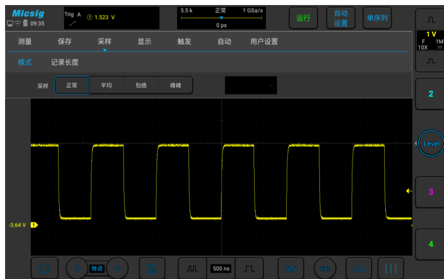
图11-5 带毛刺的正弦波，正常采样模式
