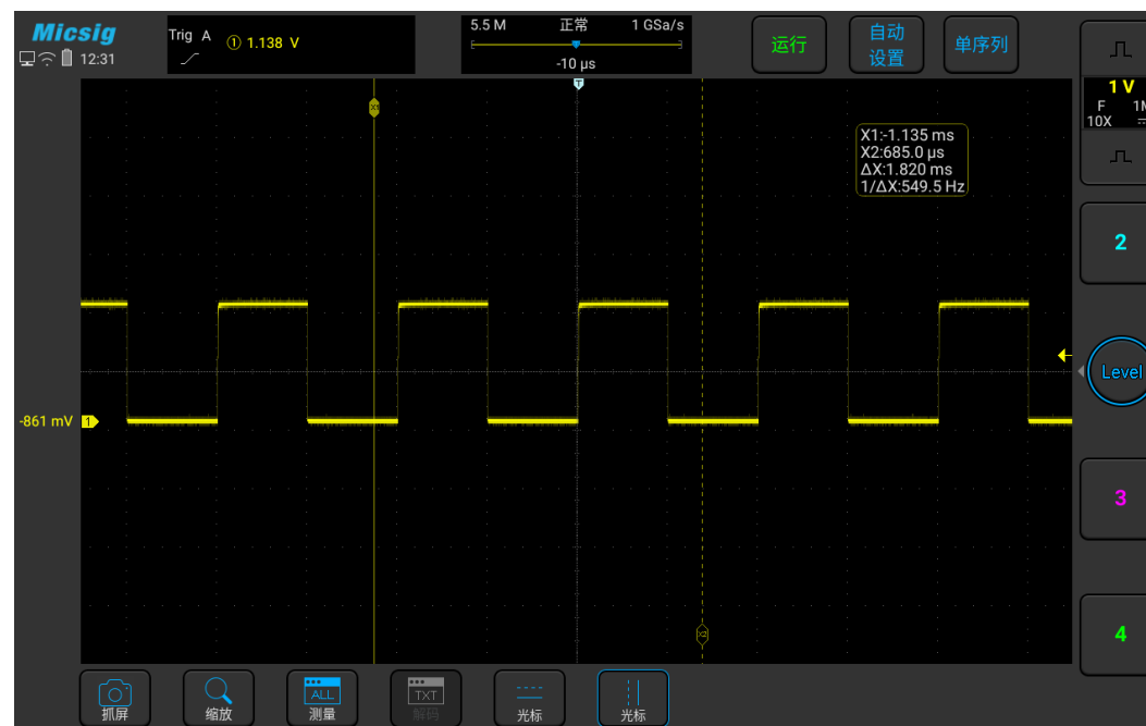
图7-12 打开光标选择框和关闭光标
