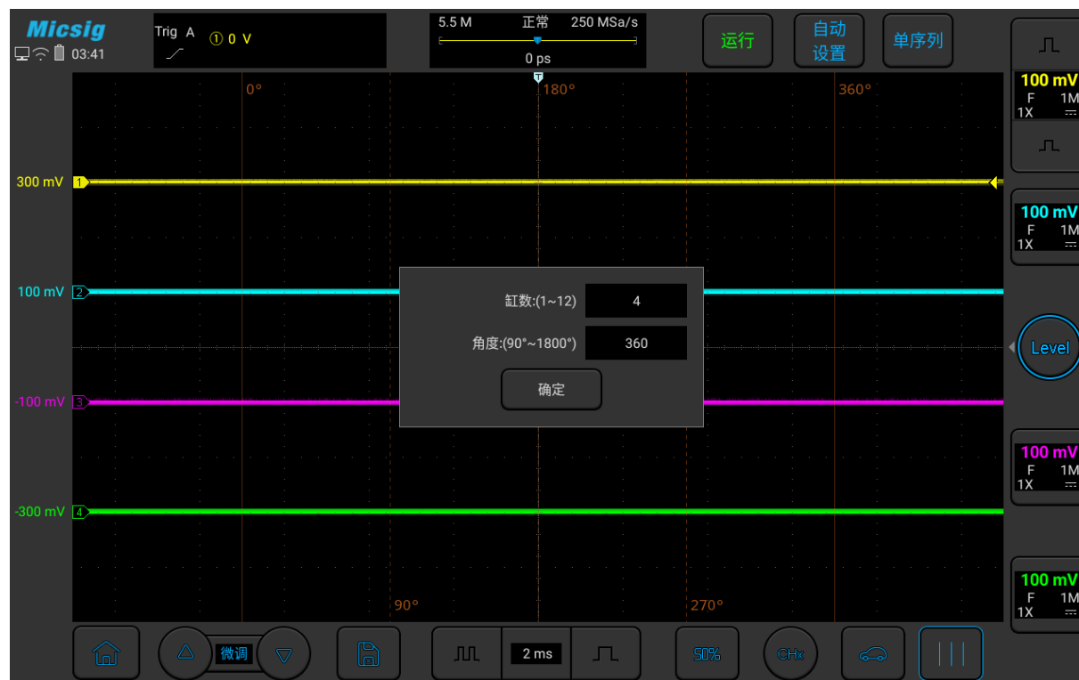
图7-15 相位标尺设置
