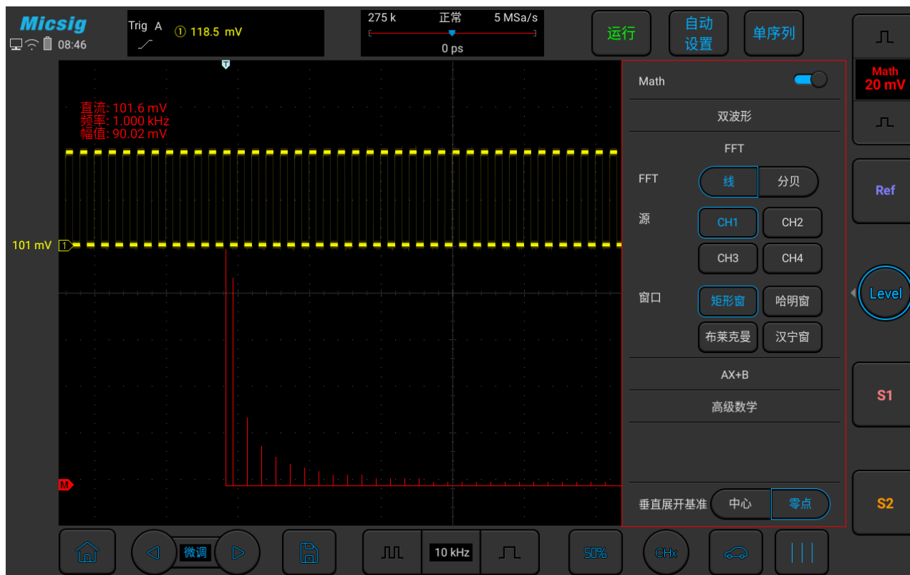
图9-3 FFT 窗口
