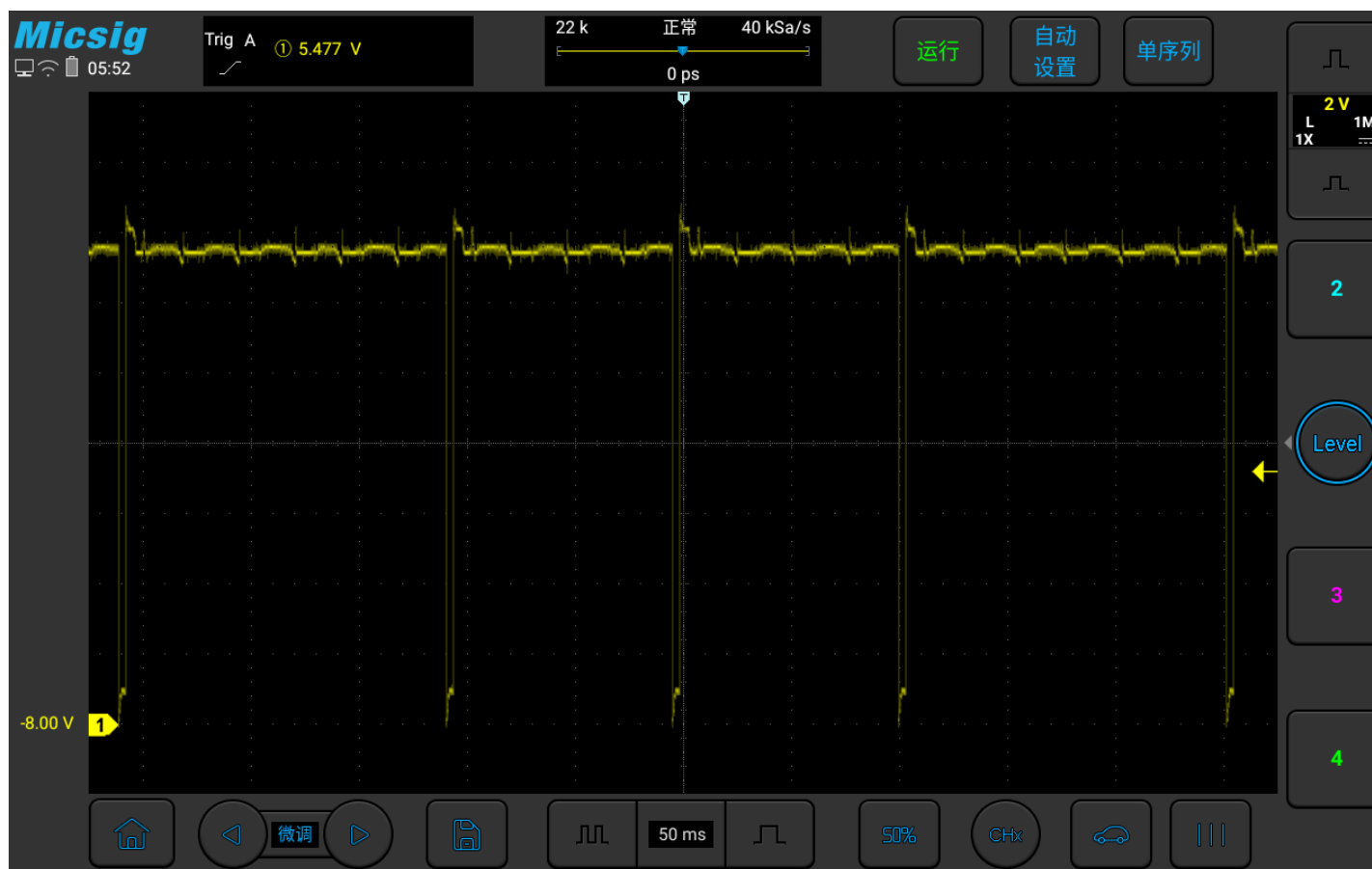
图3-30 奥迪 A6 碳罐电磁阀实测图
