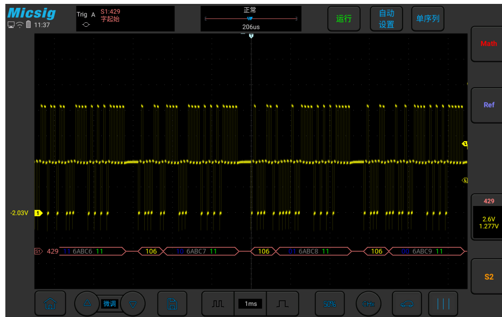
图12-28 ARINC429 图形界面
