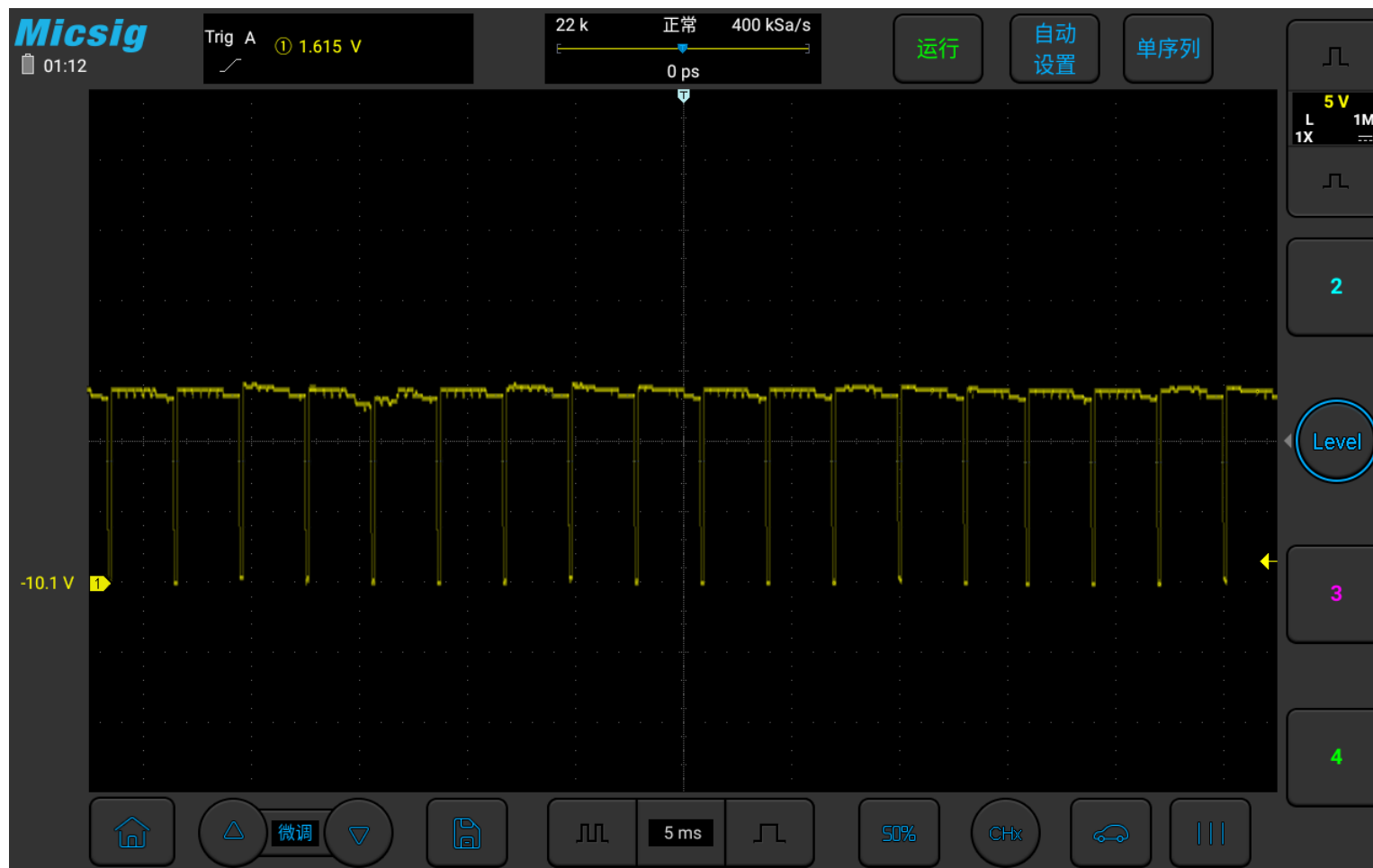
图3-43 可变气门正时实测图
