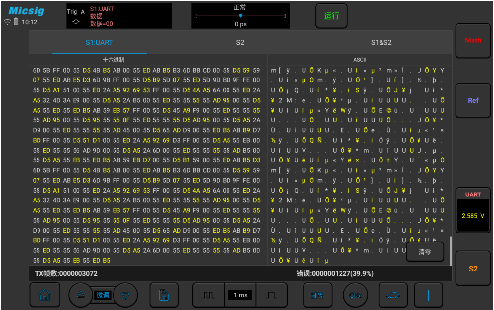
图12-2 总线解码文本模式
