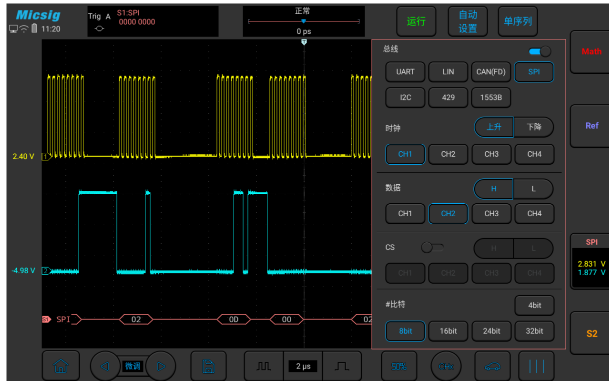
图12-18 SPI 总线配置菜单
