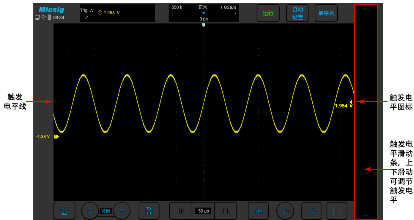
图6-8 触发电平
