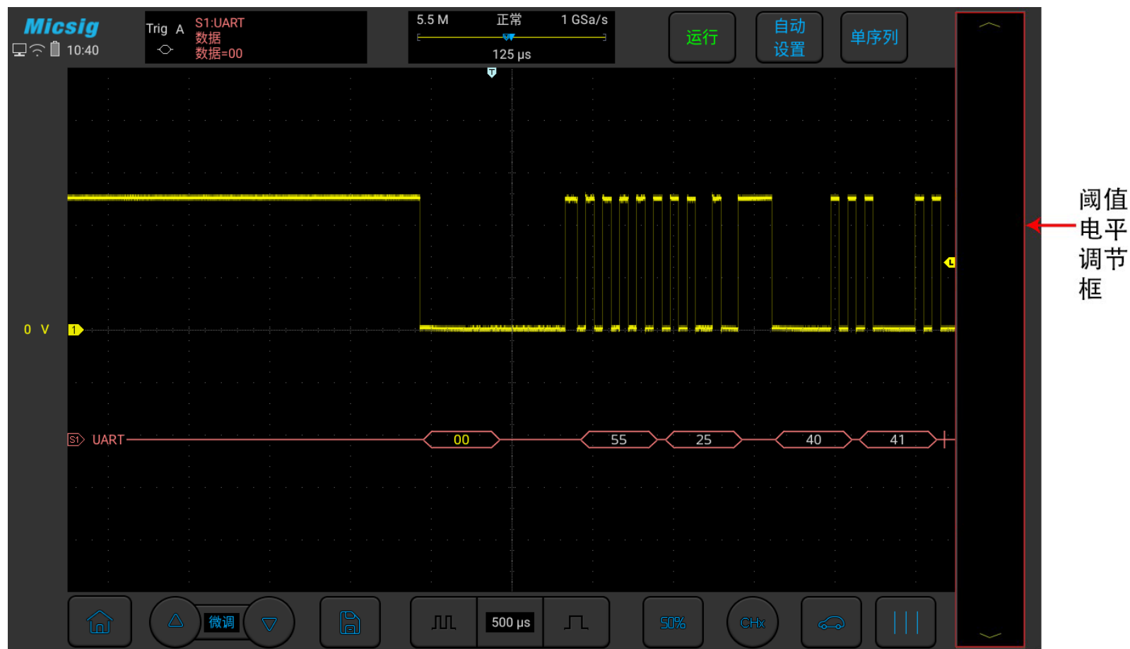
图12-7 UART 解码阈值电平调节
