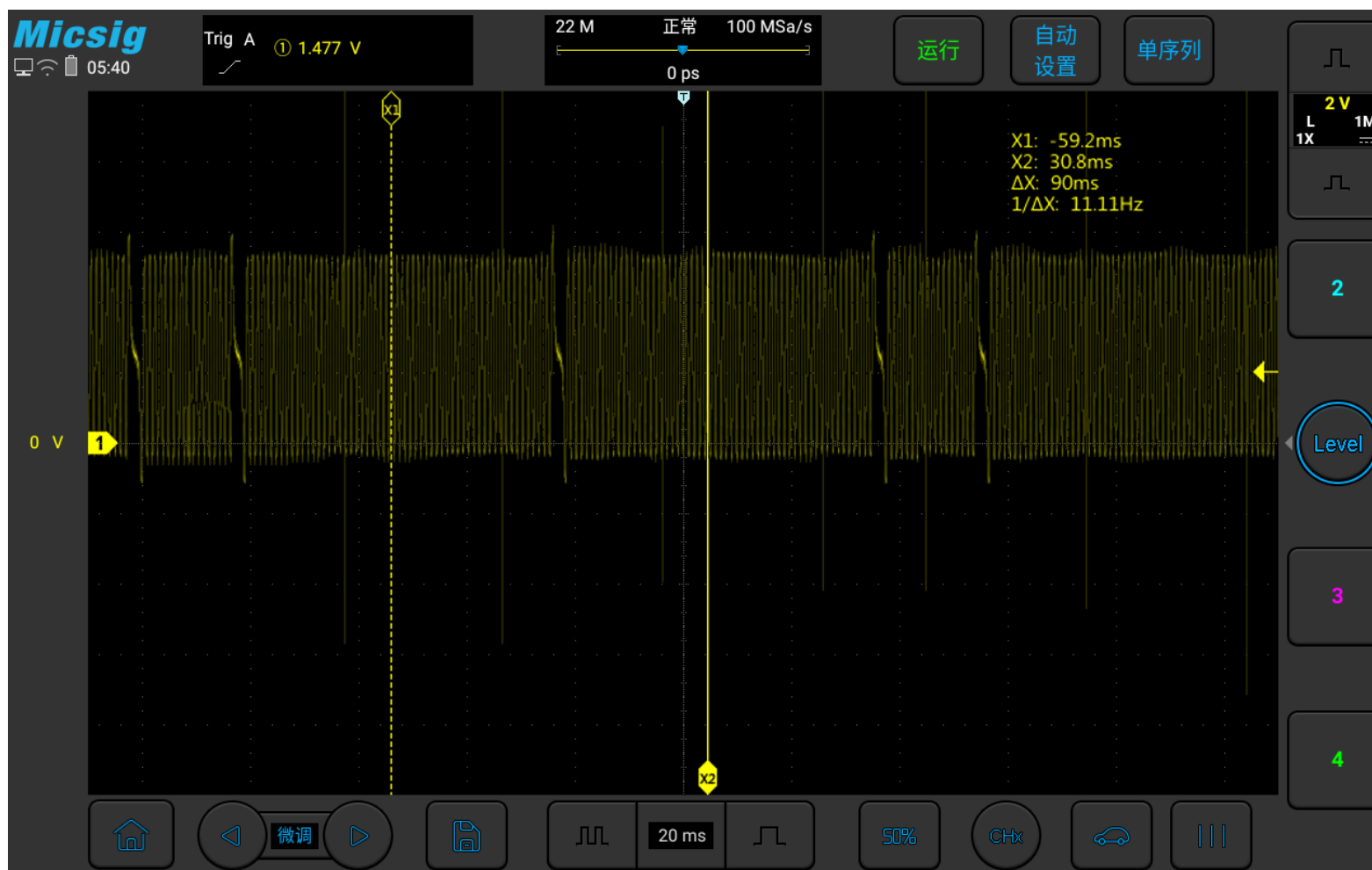
图3-18 曲轴位置传感器（感应式）的实测图
