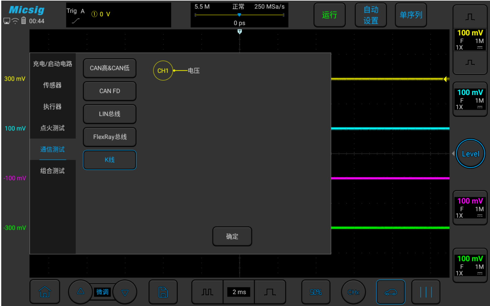
图3-54 K 线测试
