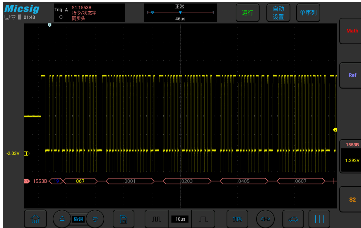
图12-32 1553B 图形界面
