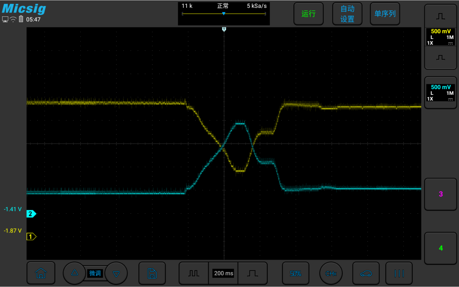
图3-28 节气门位置传感器实测图
