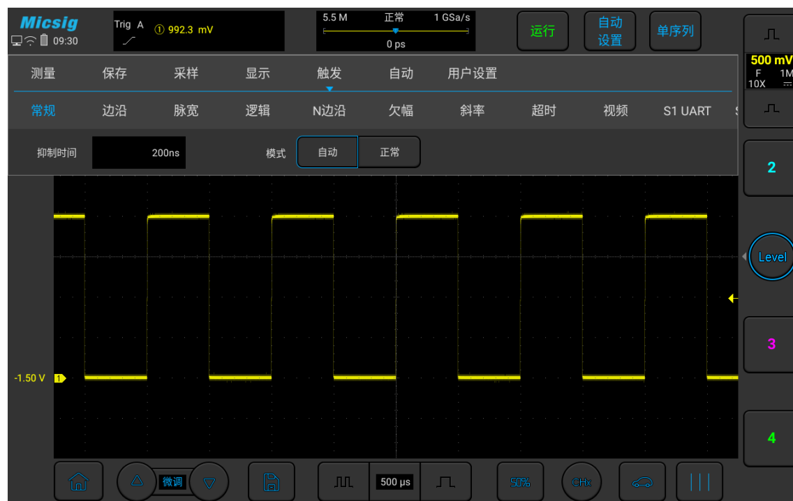
图6-5 示波器触发模式设置
