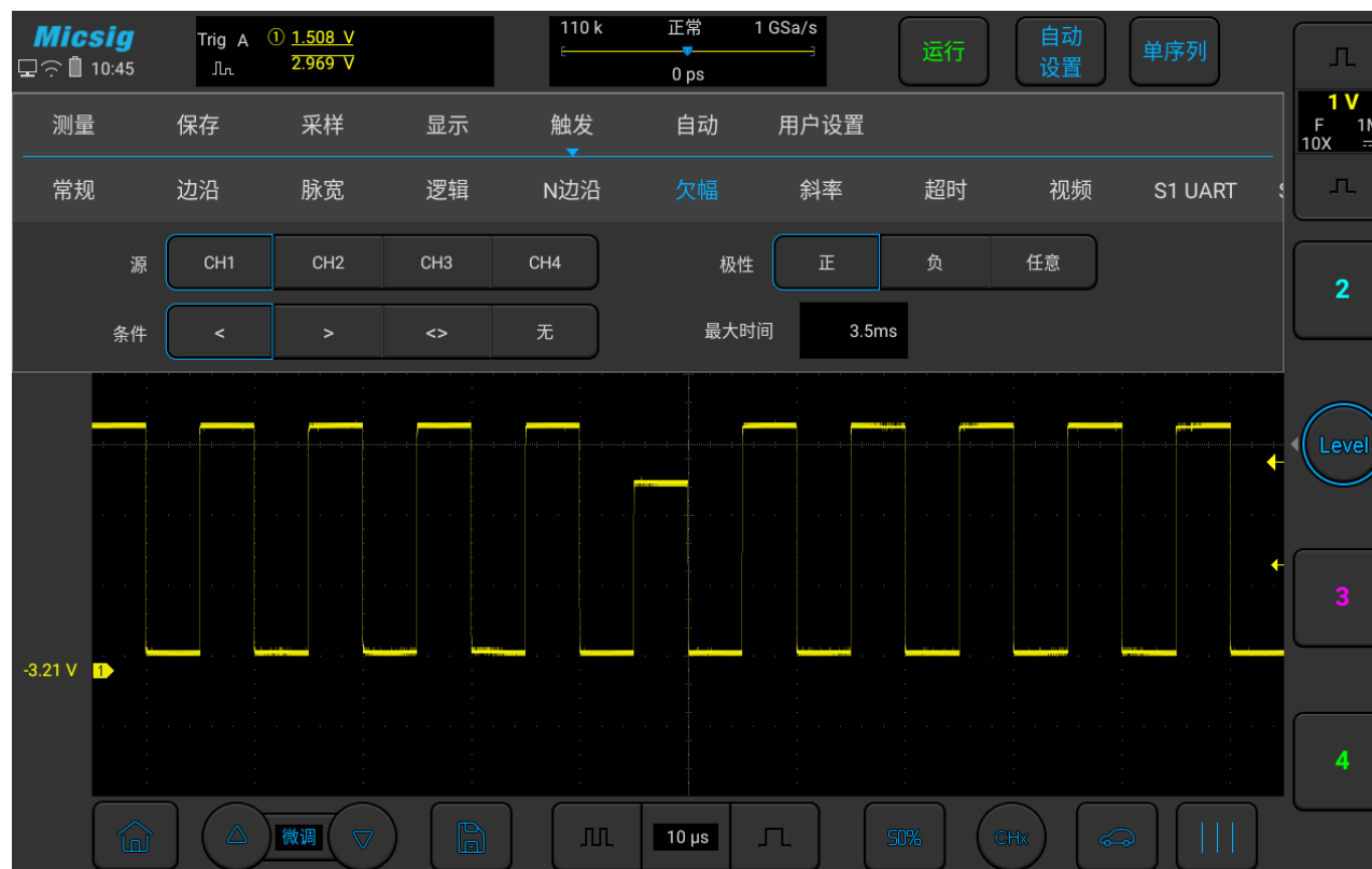
图6-25 欠幅触发设置菜单
