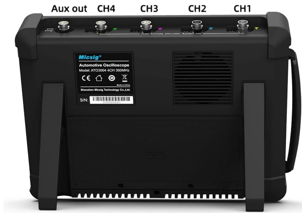
图2-3 背面
