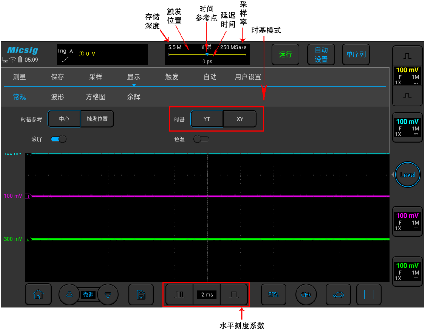
图4-1 水平系统
