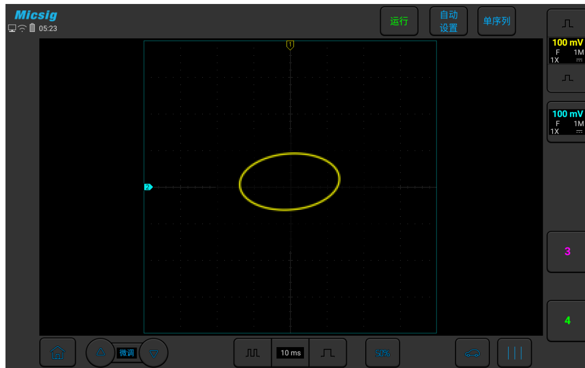
图4-8 XY 模式
