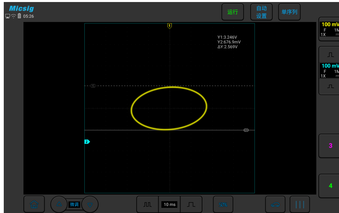
图4-10 相差测量和使用光标
