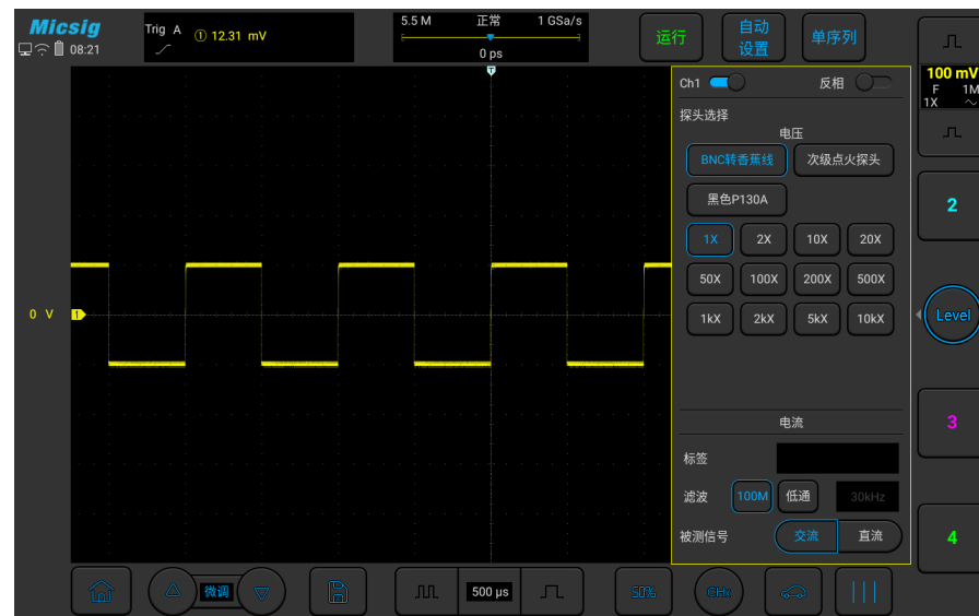
图 5-9 AC 耦合
