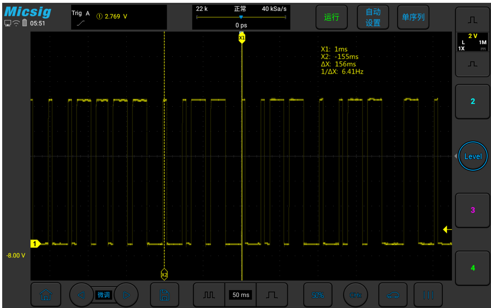
图3-15 凸轮轴位置传感器（霍尔式）实测图
