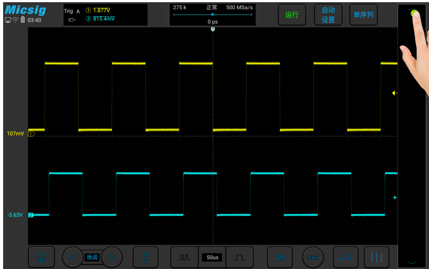
图6-22 切换触发电平通道
