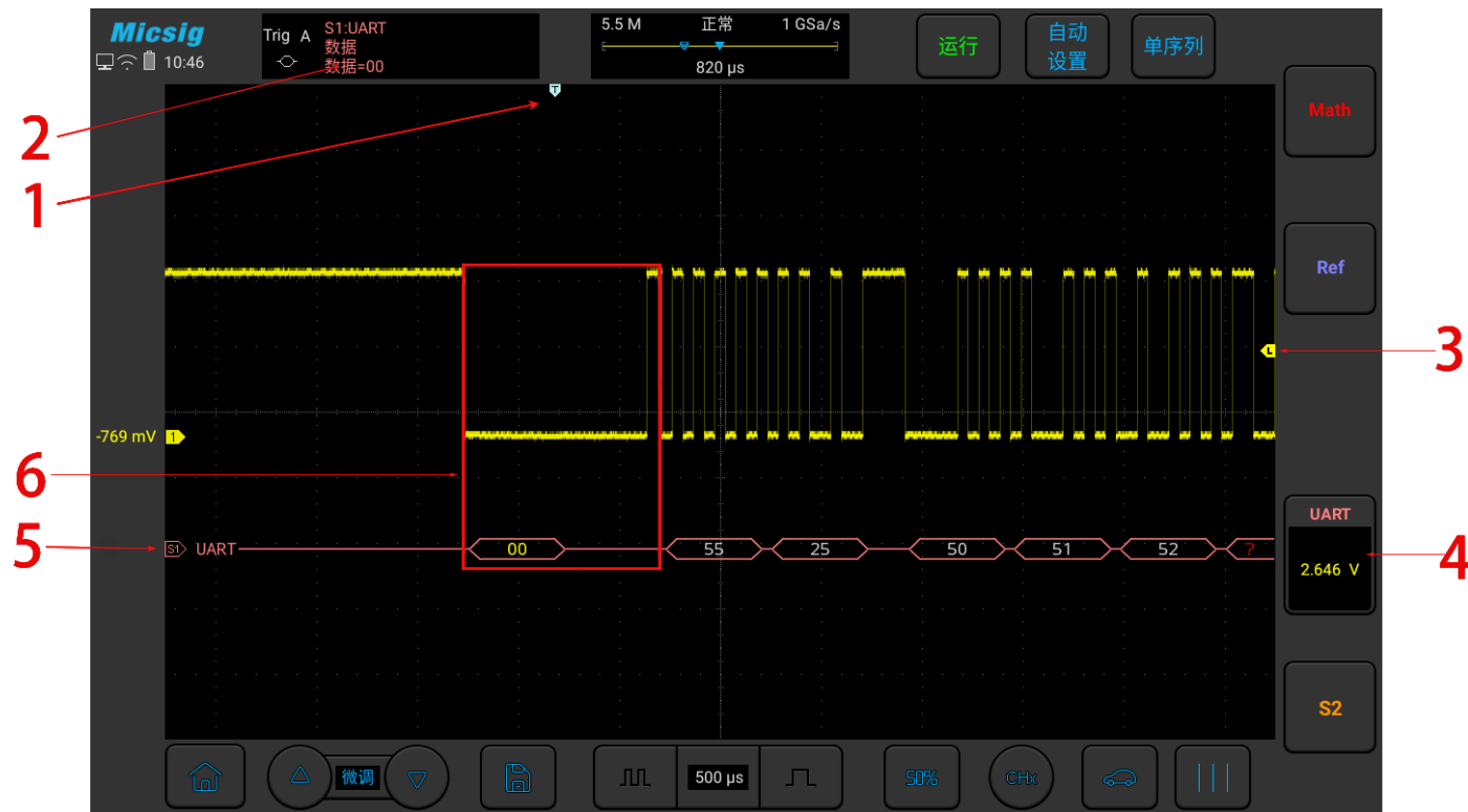
图12-8 UART 图形界面
