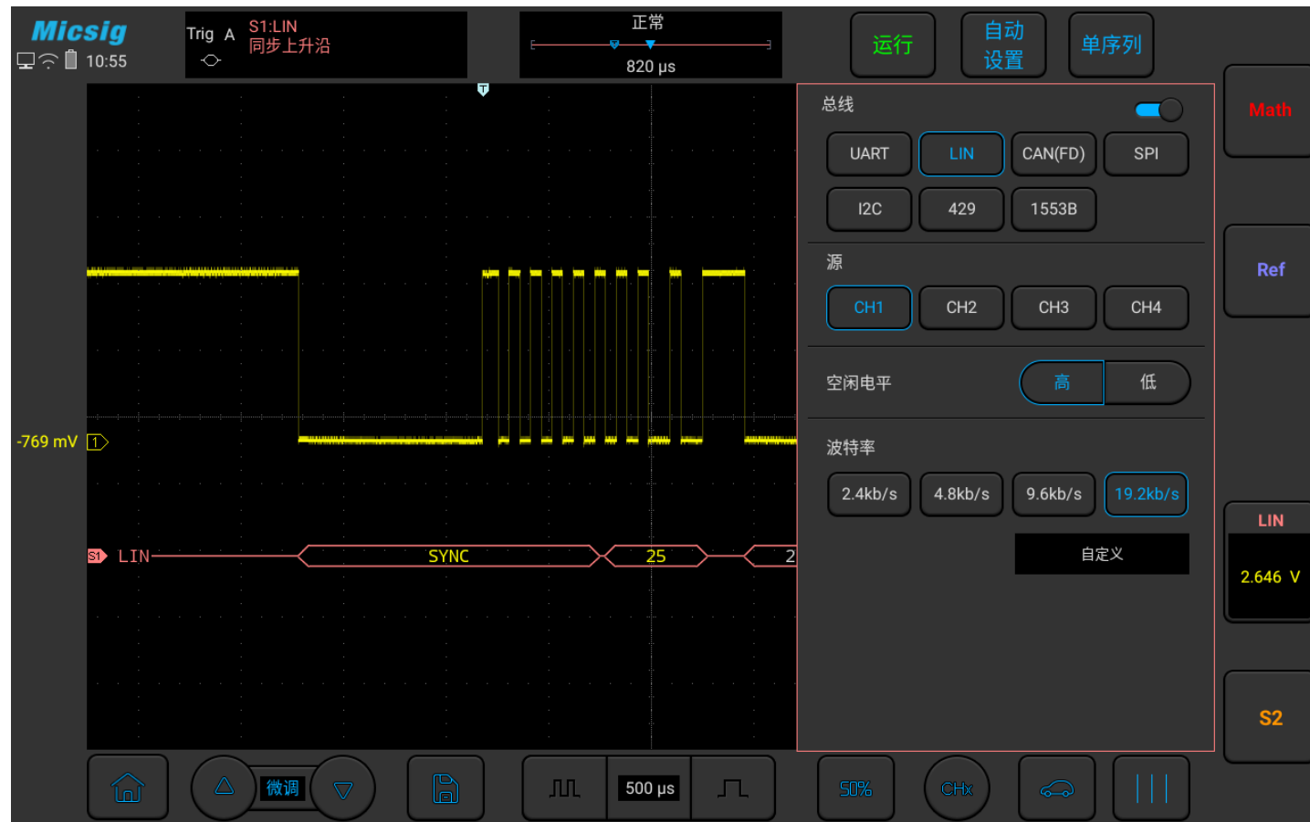
图12-10 LIN 总线配置菜单
