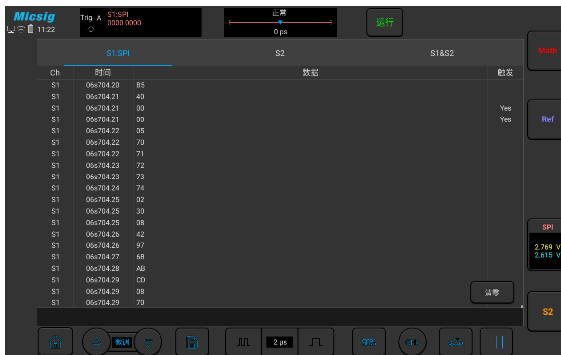
图12-21 SPI 文本界面
