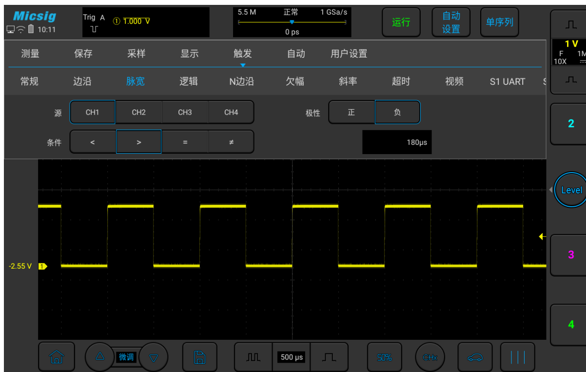
图6-15 负极性脉冲电平翻转
