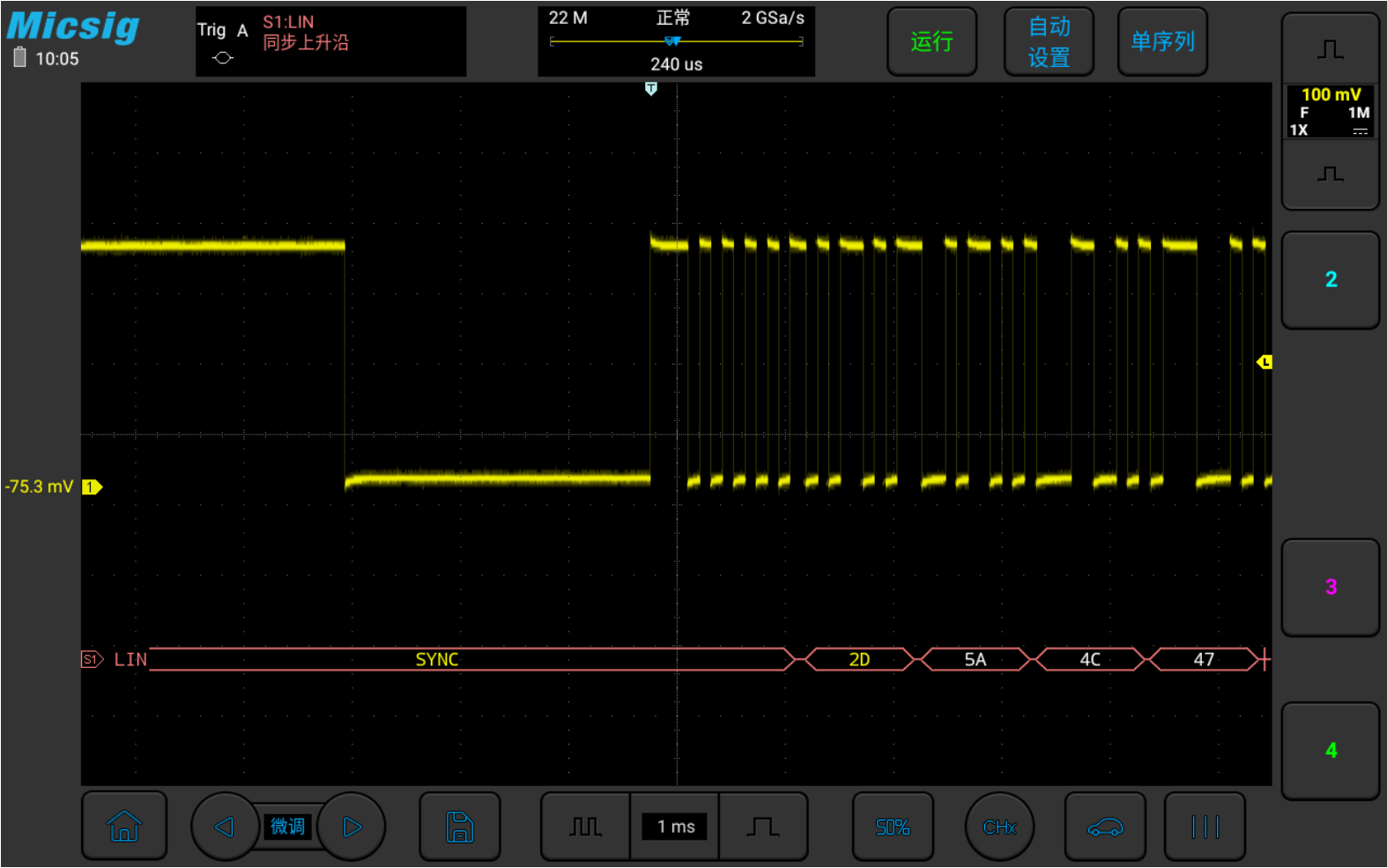
图3-52 奥迪 A6 LIN 总线实测
