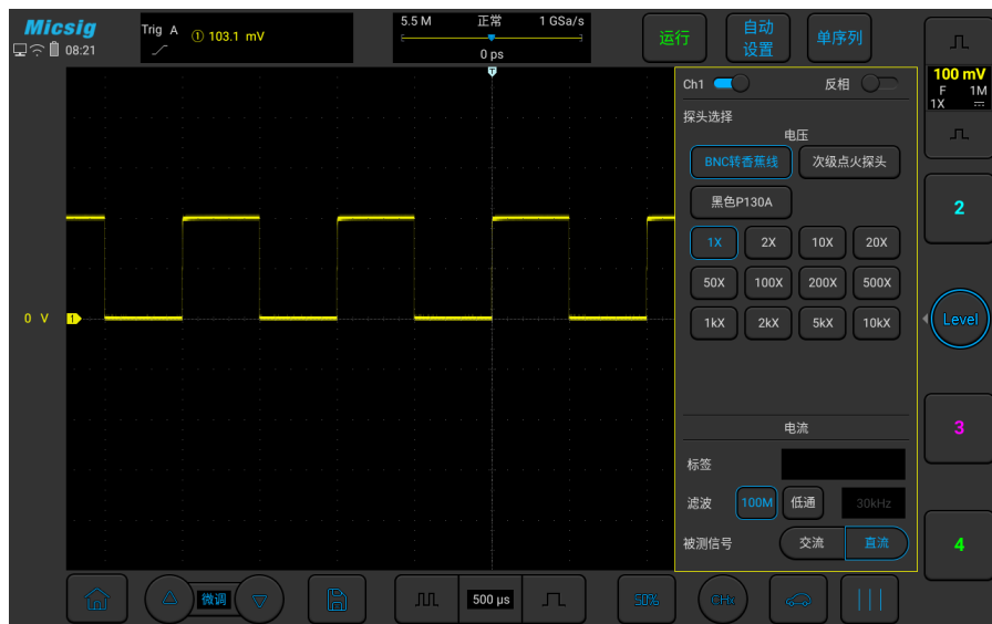
图 5-8 DC 耦合
