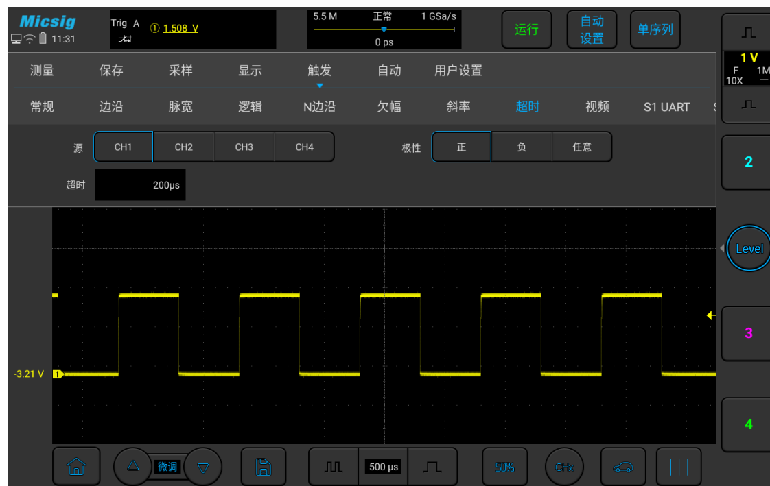
图6-29 超时触发
