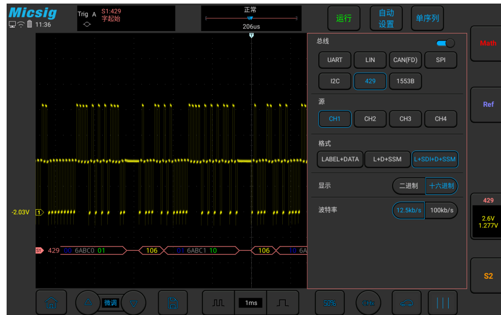
图12-26 ARINC429 总线配置菜单
