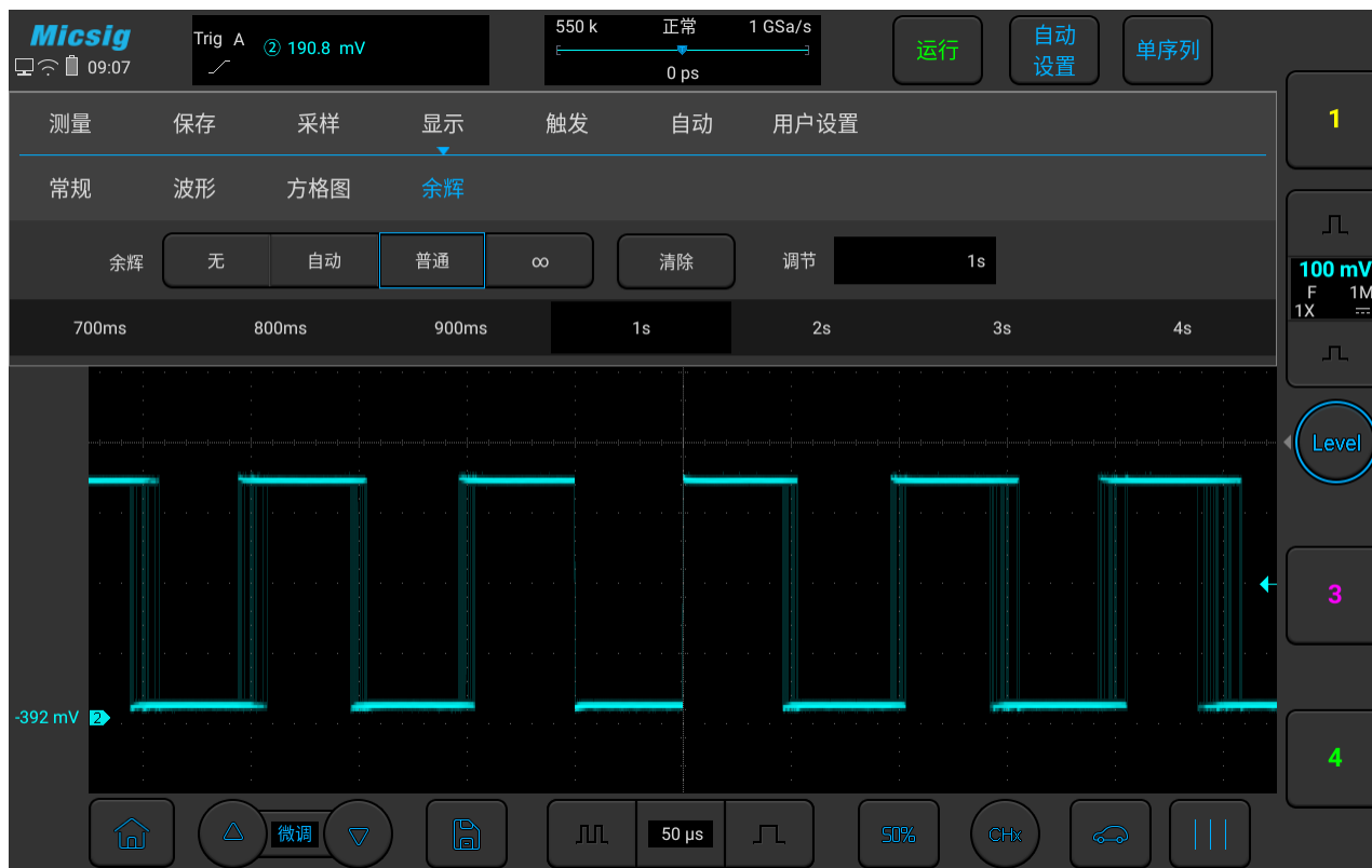
图10-4 余辉时间调节
