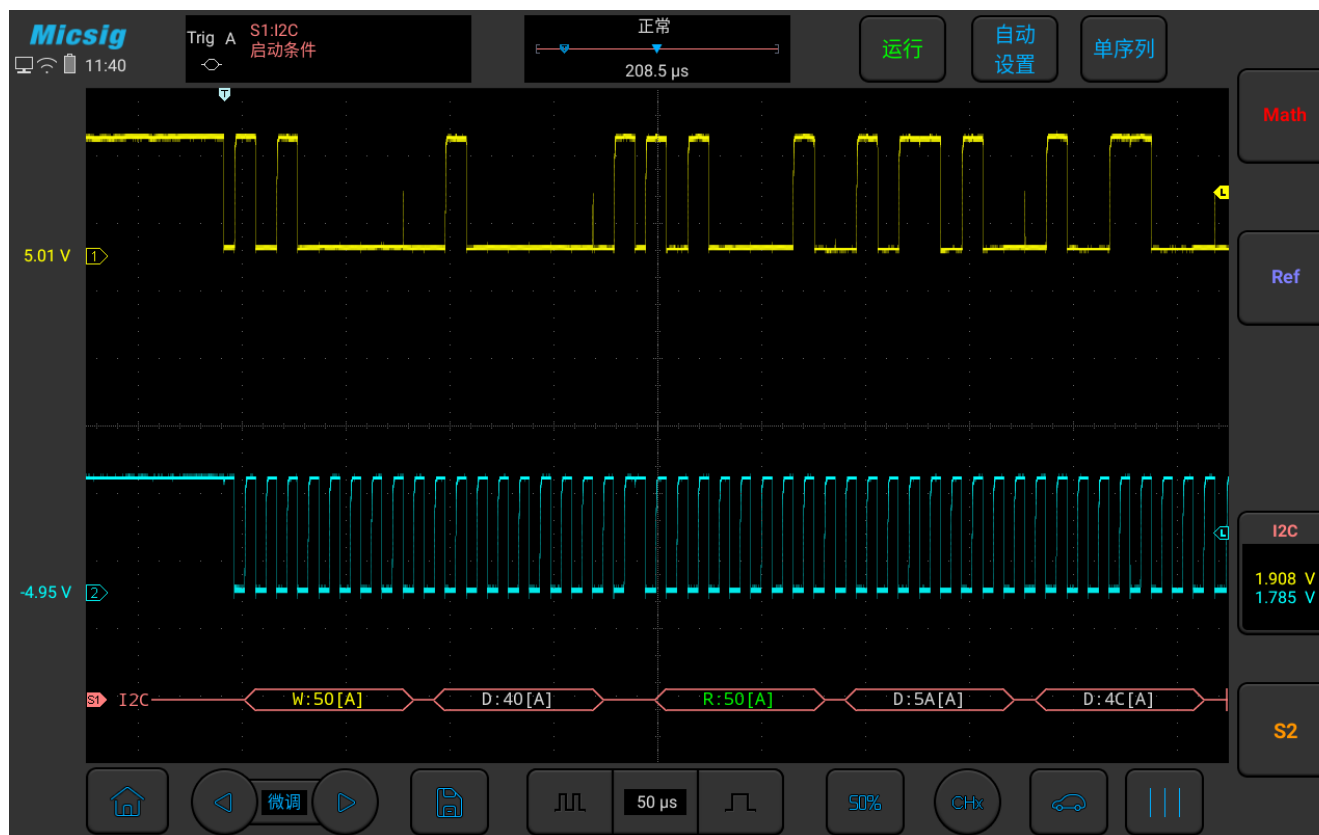
图12-24 I2C 图形界面
