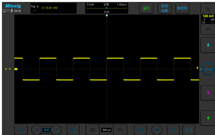
图 5-10 100M
