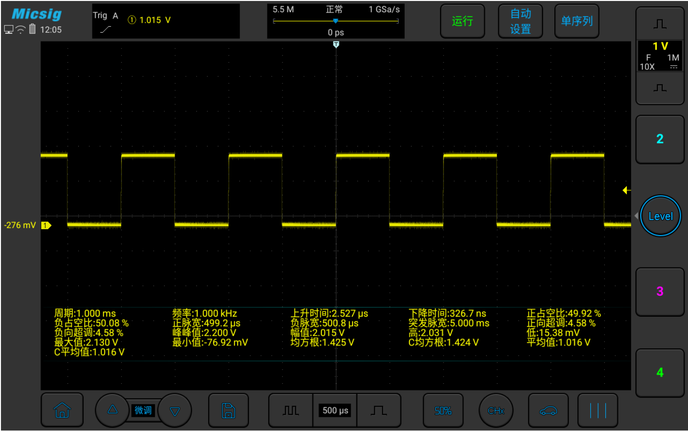
图7-3 全部测量
