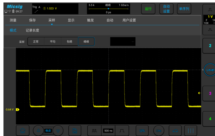
图11-6 带毛刺的正弦波，峰值采样模式
