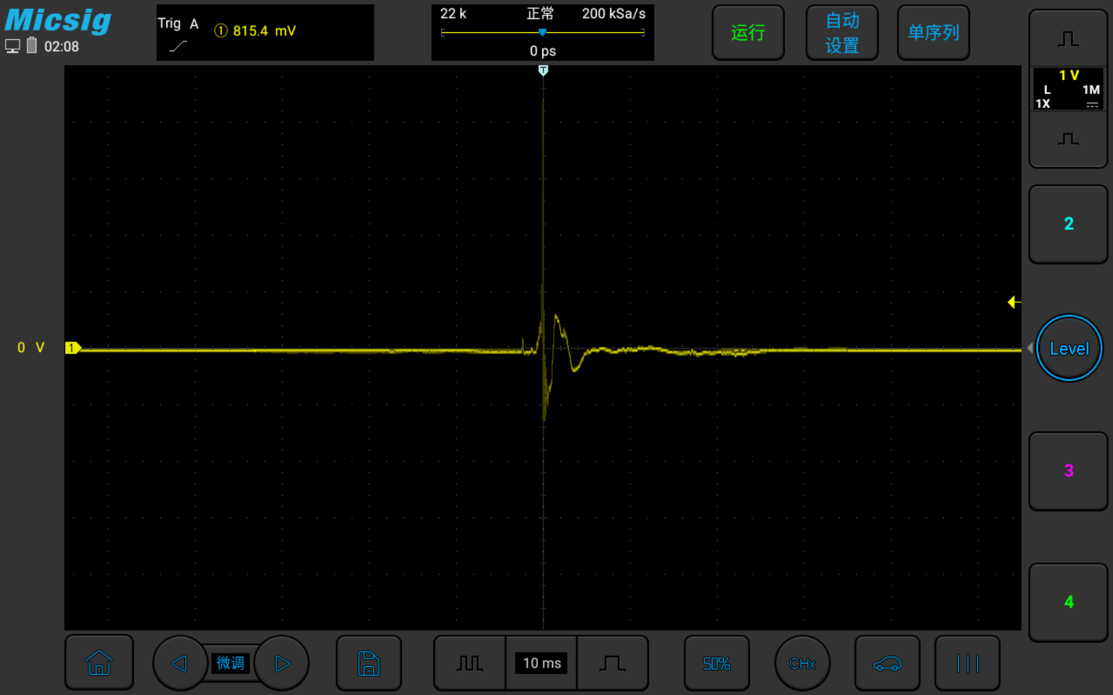
图3-22 爆震传感器实测图
