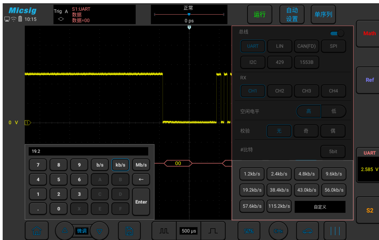
图12-5 波特率自定义设置
