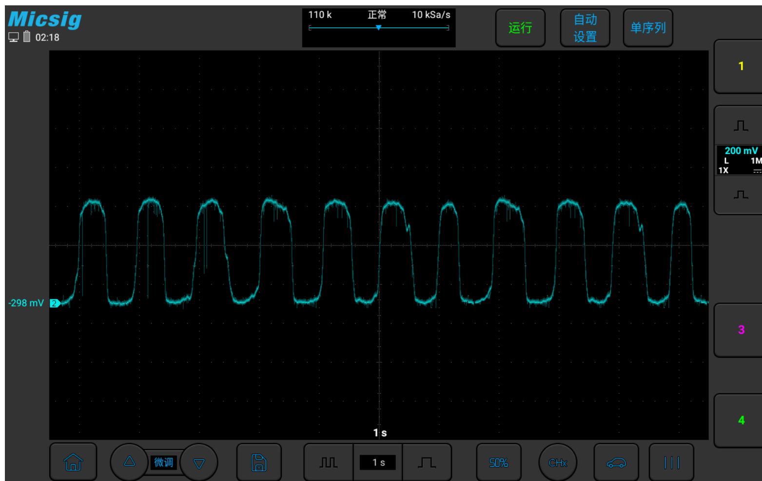
图3-24 氧传感器实测图
