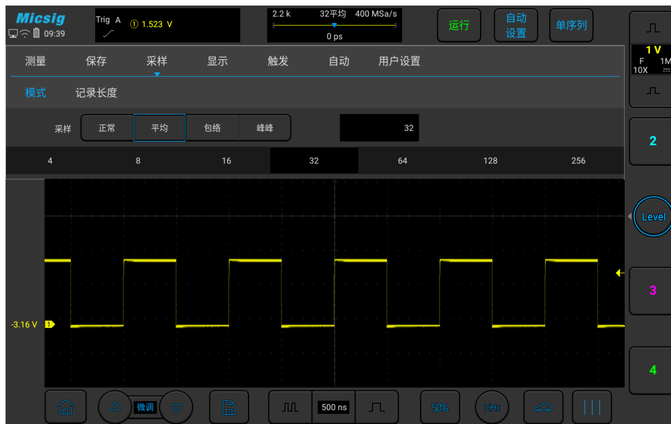
图11-7 选择平均采样模式后的波形，平均数 32
