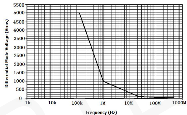
图 3: DP6700 最大差模电压 VS 频率
