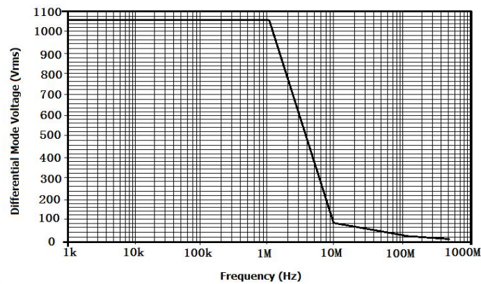
图 1: DP6150 最大差模电压 VS 频率
