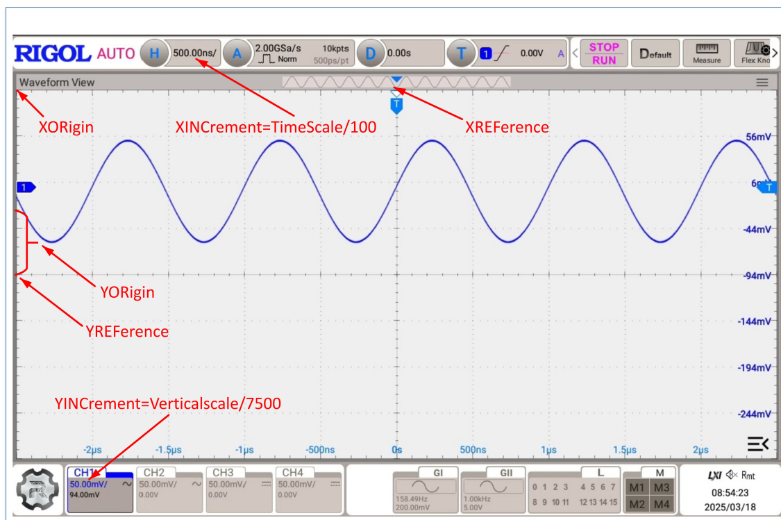
图 3.15 NORMAL 模式下的参数定义
