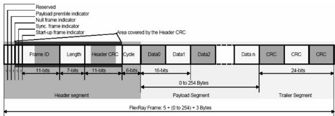
图 3.13 FlexRay 总线帧格式
