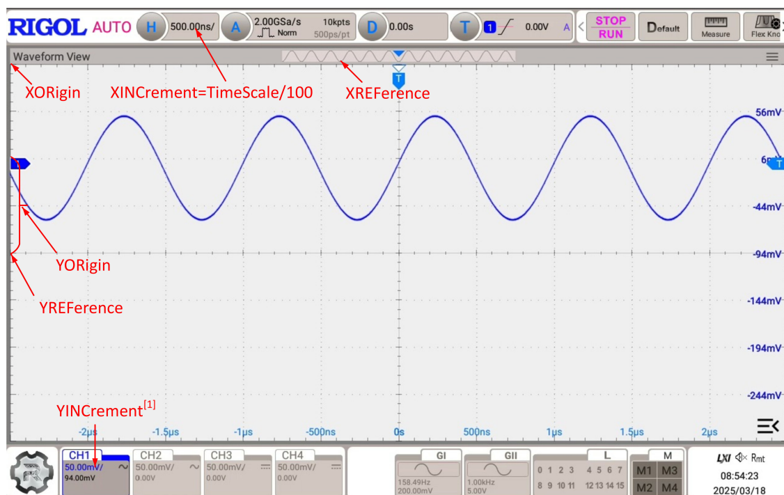
图 3.16 RAW 模式下的参数定义
