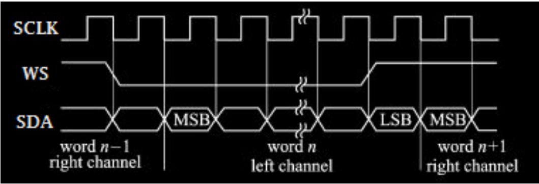
图 3.12 I2S 总线时序图
