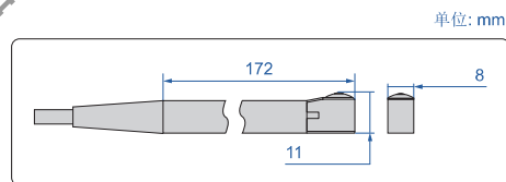
FE90探头尺寸
