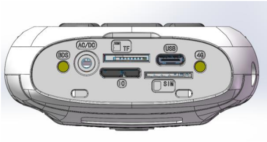
图 4-1-4 底部接口
