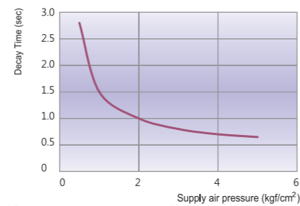
供应气体压力和除电性能特性图
