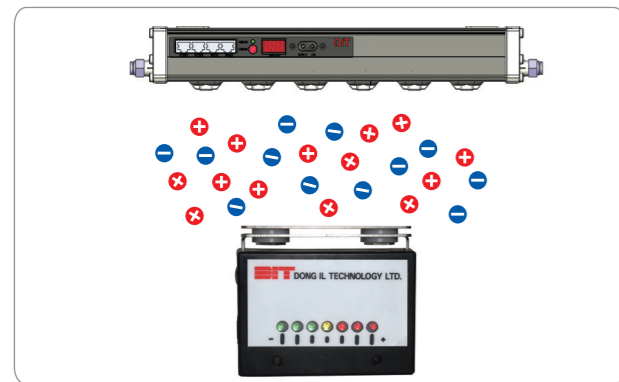
离子发生器下端, 产品通过的距离测量离子平衡度的偏向与否
