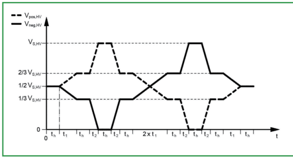
高压电压偏移测试的测试步骤1的高压电压曲线
