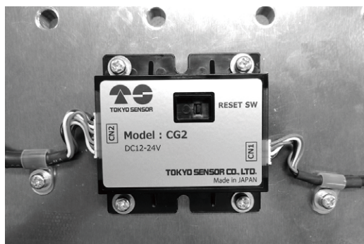
主体安装例
