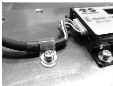
电缆固定例
