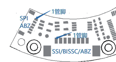
连接器及引脚1位置
