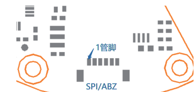
6芯连接器及引脚1位置
