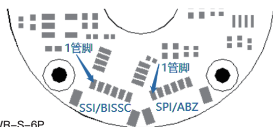
连接器及针脚1位置
