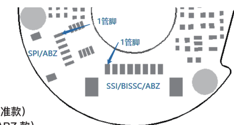
连接器及针脚1位置
