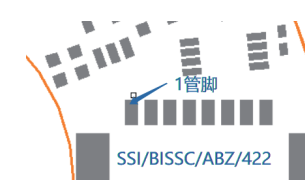
8芯连接器及引脚1位置
