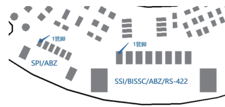
连接器及引脚1位置
