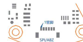
6芯连接器及引脚1位置
