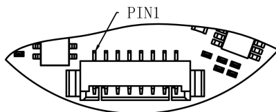
连接器及针脚 1 定义
