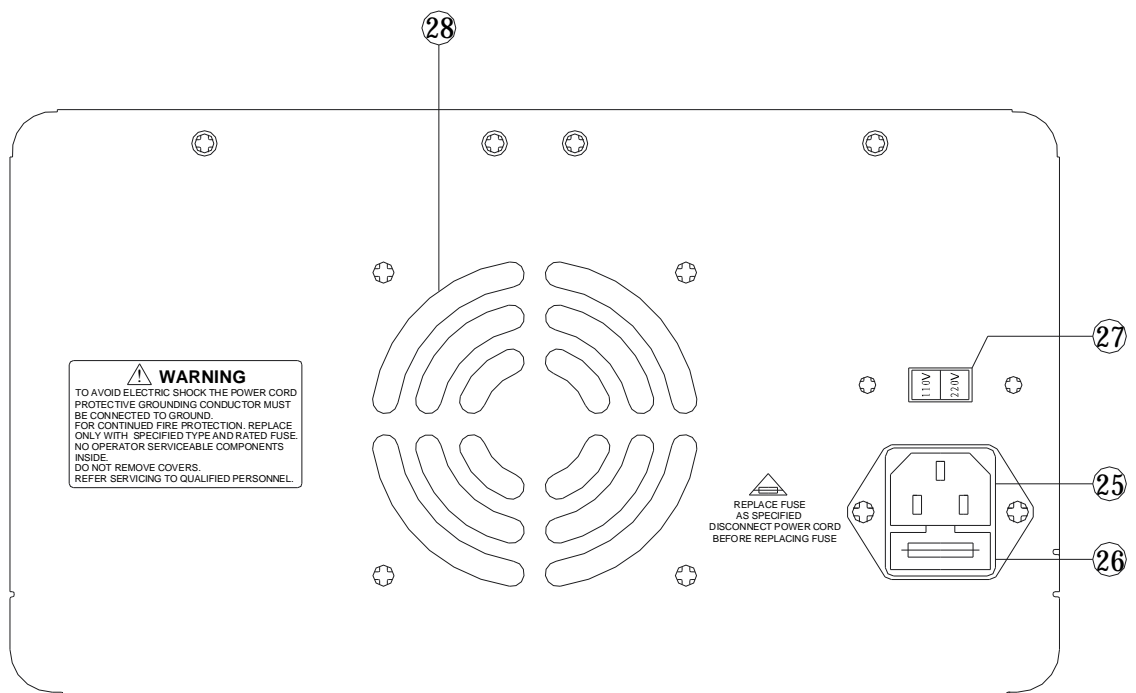
● 图 3-2 后面板
