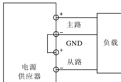
正/负双电源串联模式
