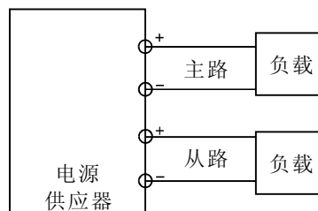
独立模式
