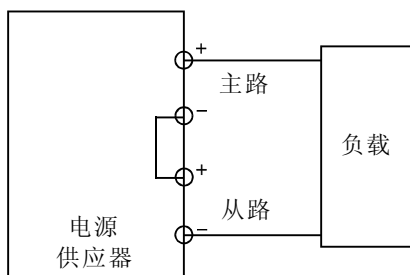
单电源串联模式
