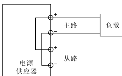
并联模式
