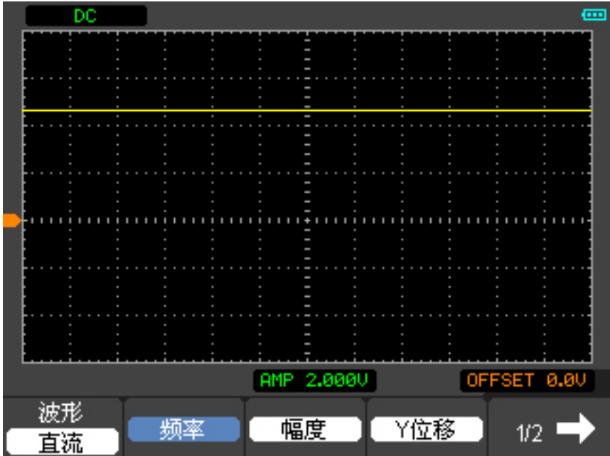
图 5-14 直流波形
