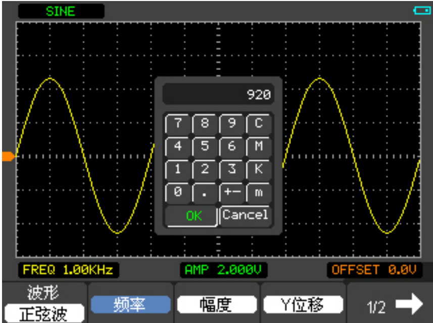
图 5-3 键盘窗口
