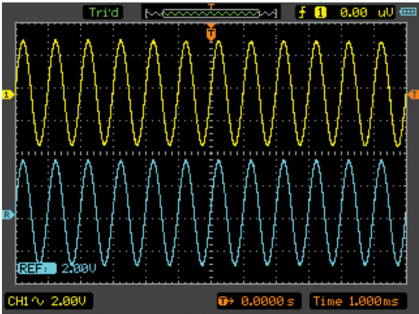
图 2-17 REF 显示
