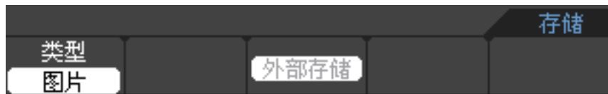
图 2-33 位图菜单
