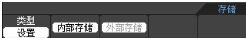
图 2-32 配置菜单
