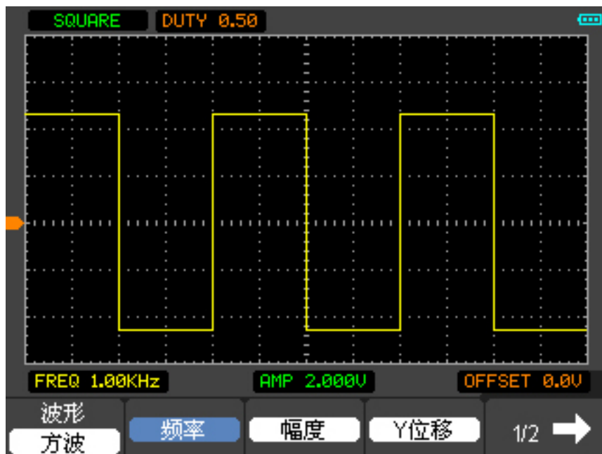
图 5-5 方波
