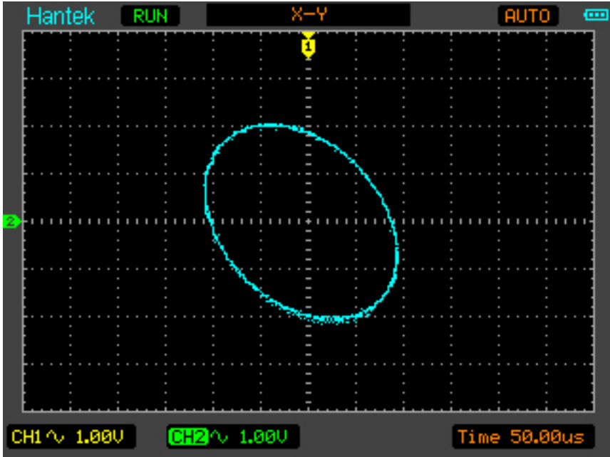
图 3-2 李沙育图
