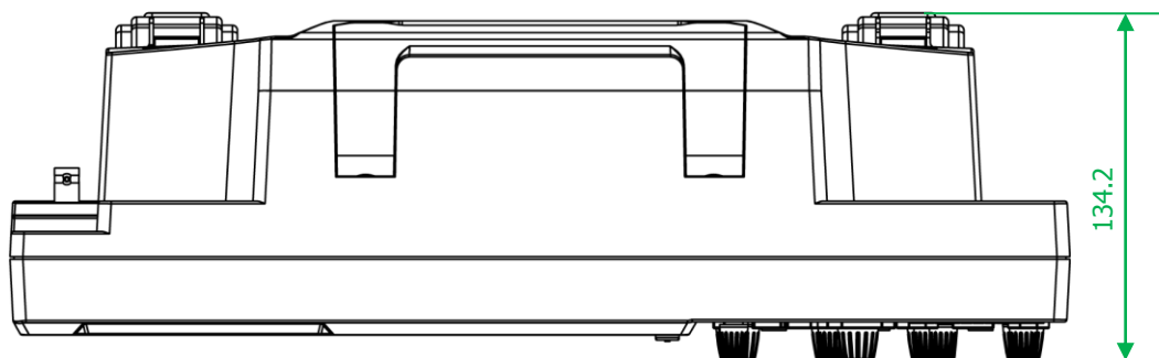
图 1-2 俯视图
