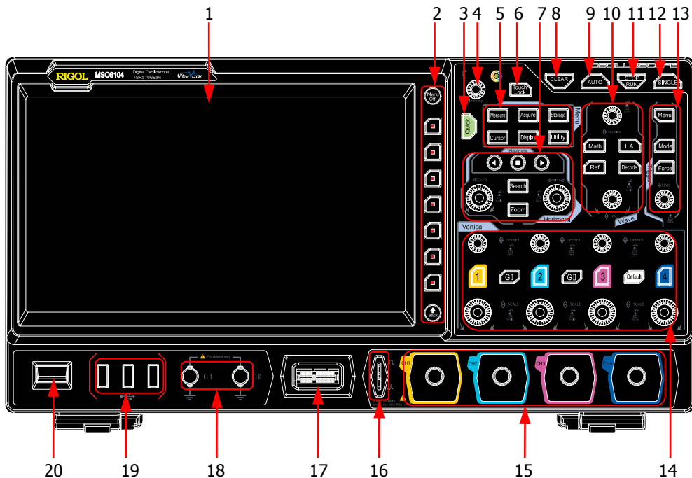
图 1-13 前面板总览
