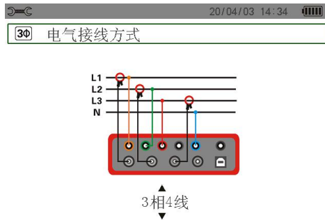
图 4-6 三相 4 线连接
