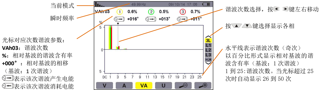
图 7-6 视在功率谐波 3L 显示
