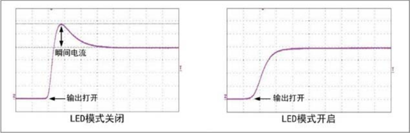
LED模式打开时, 电流与电力对应关系
