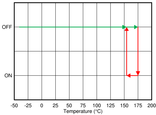
图 6-35. Thermal Shutdown
