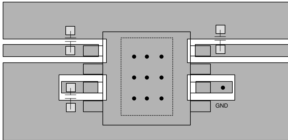
图 10-1. DDA Package Fixed Output
