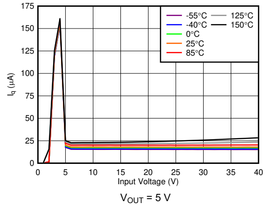
图 6-26. Quiescent Current ( I_Q ) vs V_{IN}
