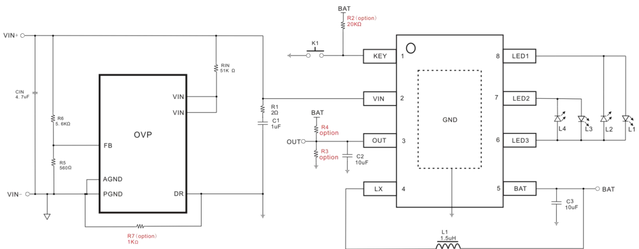
Fig2.带 OVP 应用电路
