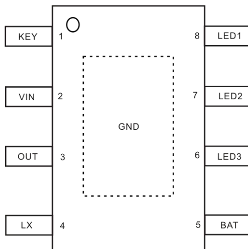
Fig3.管脚示意图
