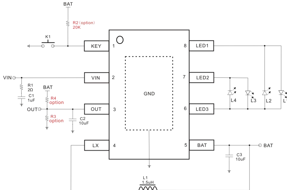
Fig1.CP6294D 典型应用电路
