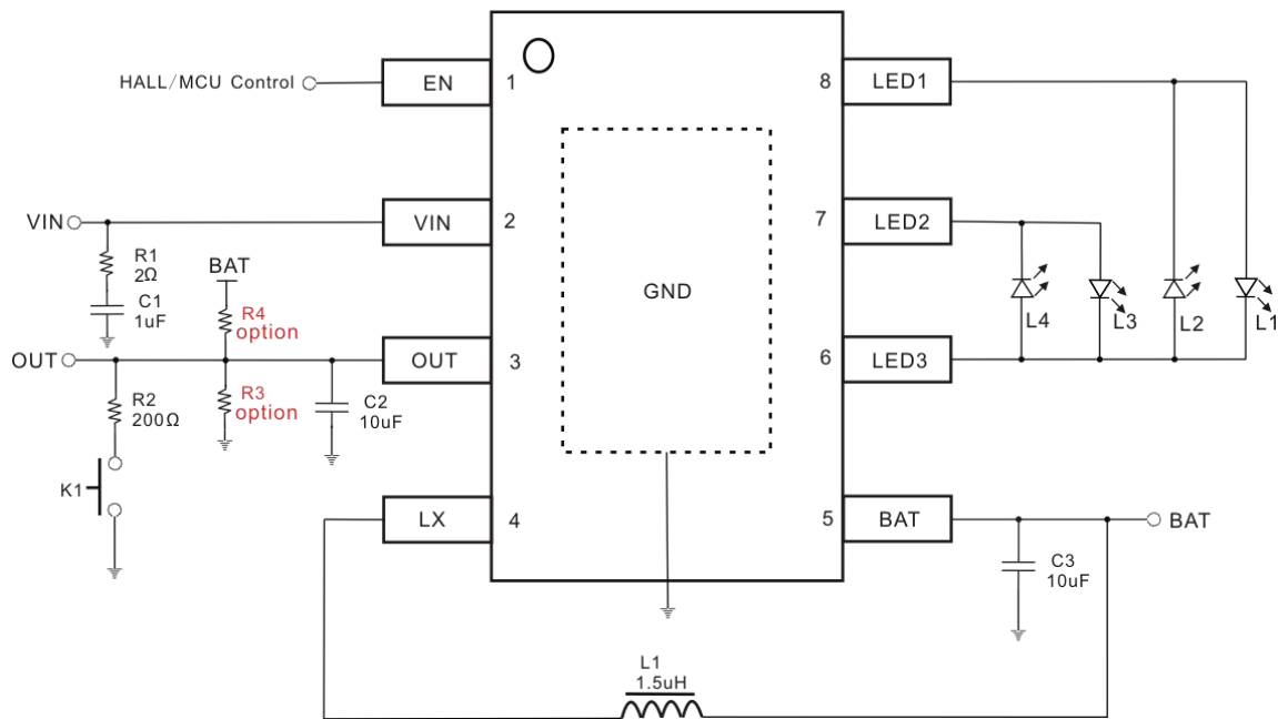
Fig1.CP6294EB 典型应用电路
