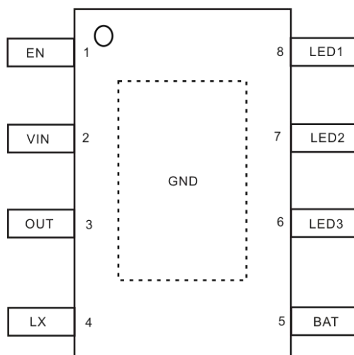
Fig3.管脚示意图
