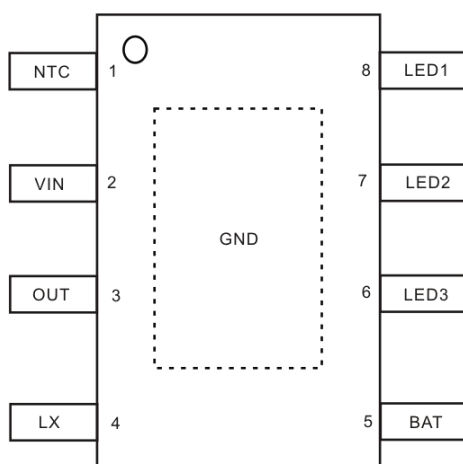
Fig3.管脚示意图
