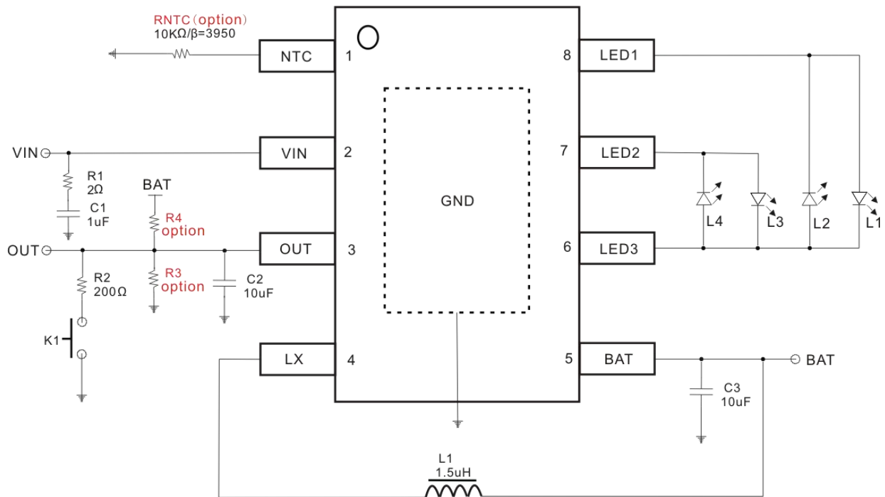
Fig1.CP6294TB 典型应用电路
