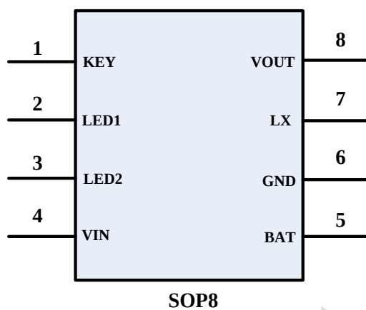
图 2 IP5413 引脚图
