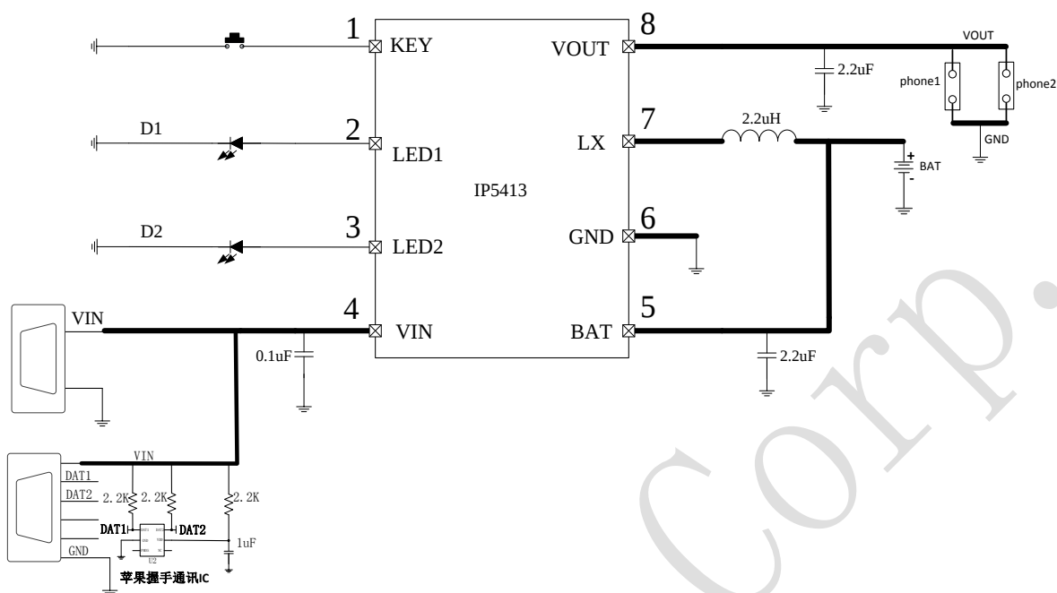
图 10 2LED 电量显示典型应用原理图
