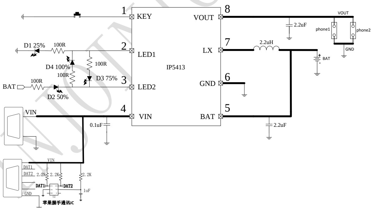
图 11 4LED 电量显示典型应用原理图
