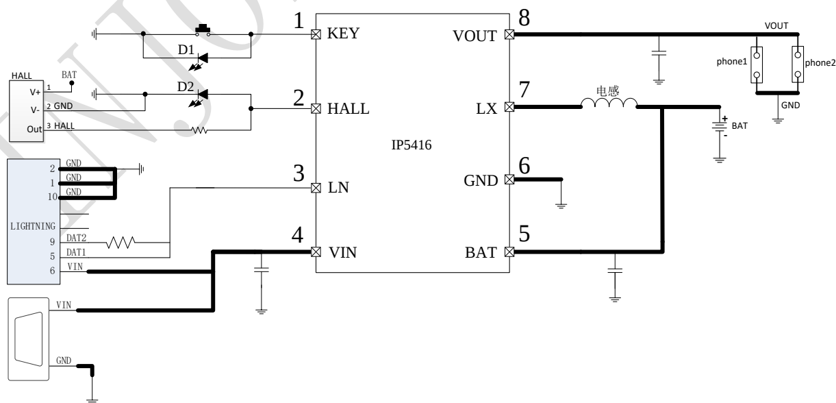
图 1 IP5416 简化应用原理图
