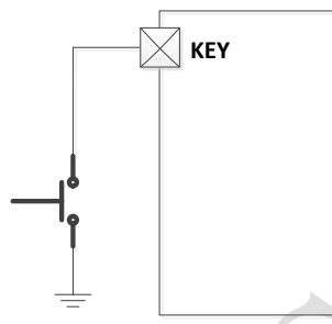
图 8 IP5416 KEY 电路图
