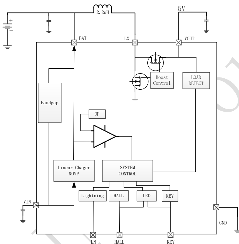
图 3 IP5416 内部系统框图
