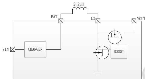
图 6 IP5416 路径管理示意图
