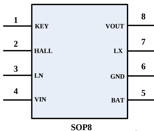
图 2 IP5416 引脚图
