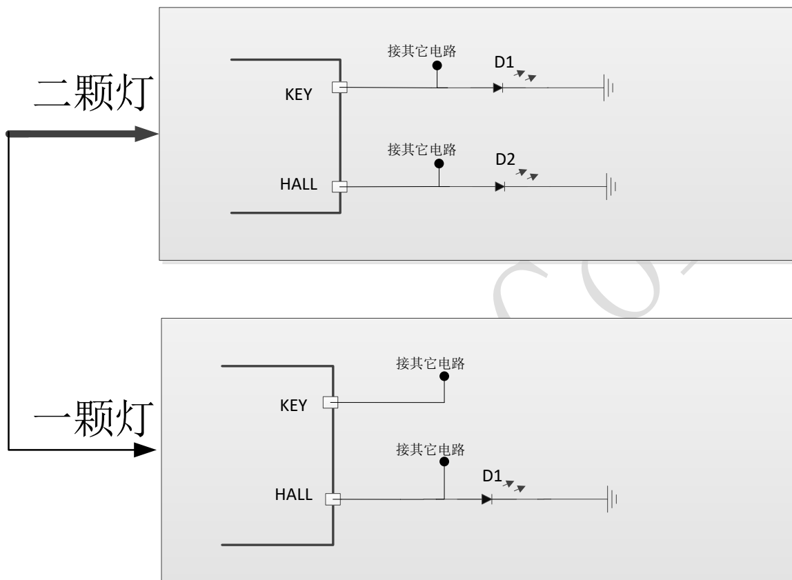
图 7 LED 显示配置电路图
