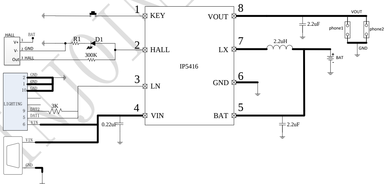
图 11 1LED 电量显示典型应用原理图
