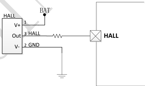
图 9 IP5416 HALL 电路图
