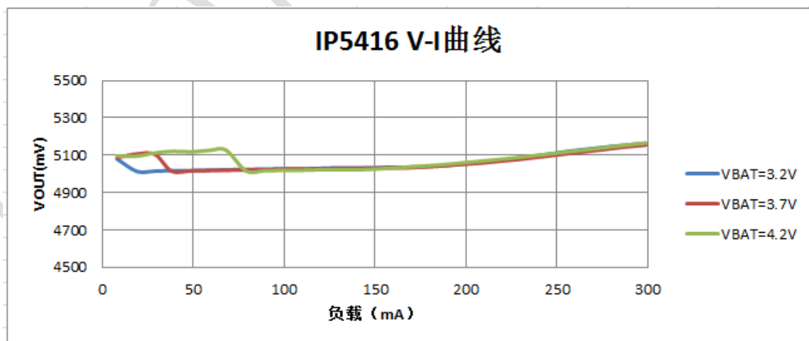
图 5 IP5416 V-I 曲线图
