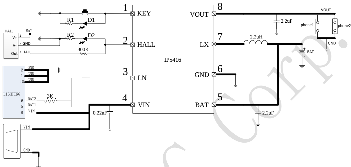
图 10 2LED 电量显示典型应用原理图
