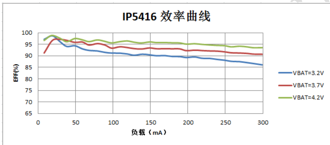
图 4 IP5416 升压效率图
