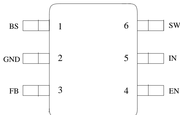
SOT23-6 (CP3471)
