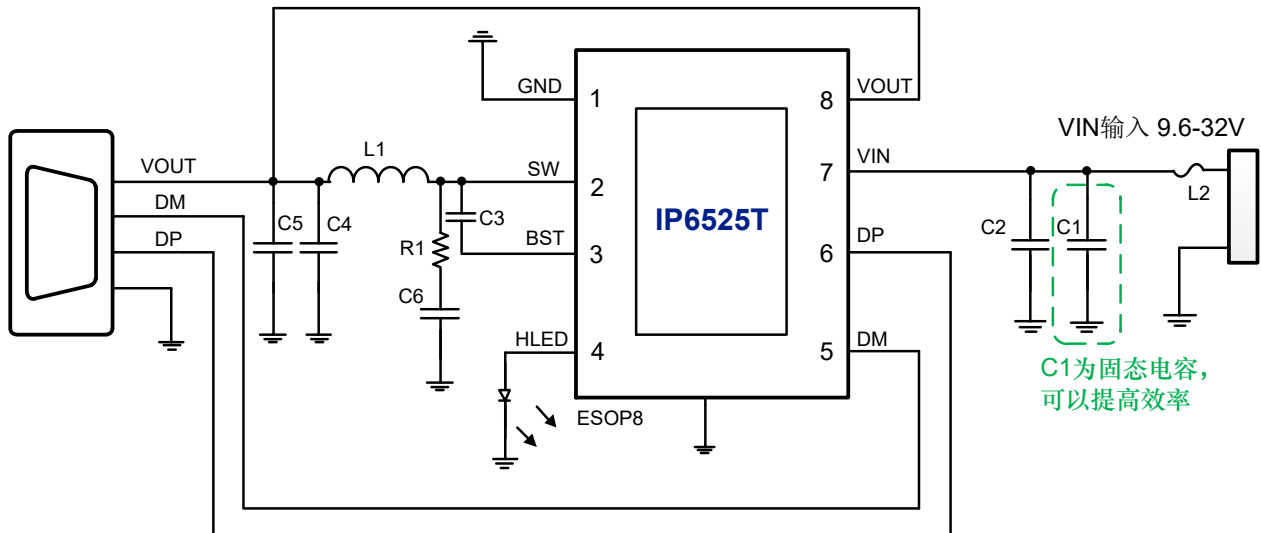
图 5 IP6525T 输出应用原理图
