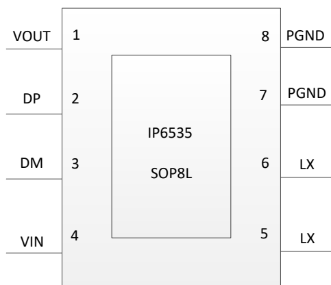
图 1 IP6535 引脚图
