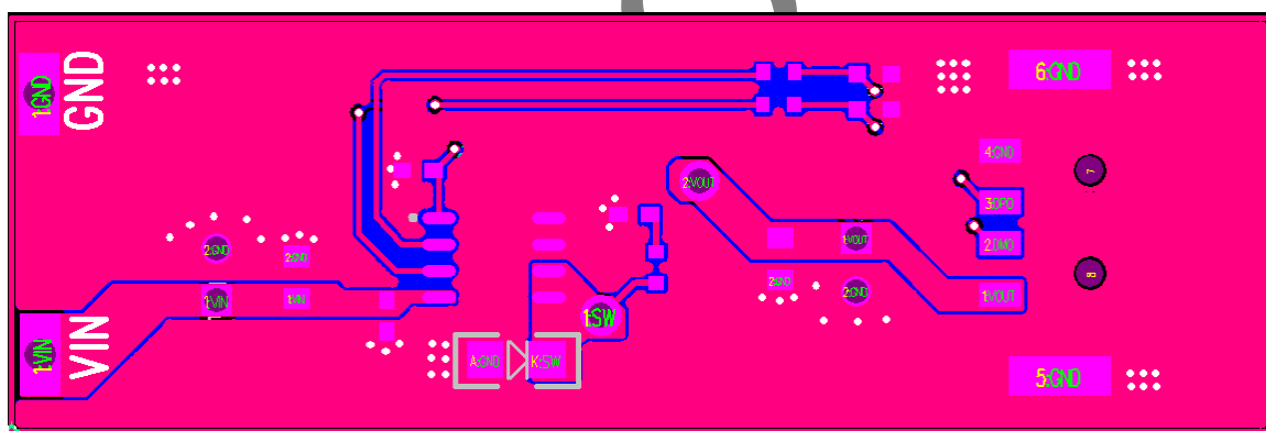
图 3 IP6535 demo 板
