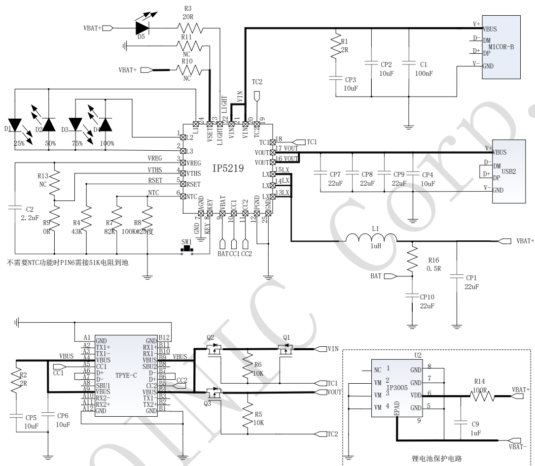
图 6 4LED 电量显示典型应用原理图
