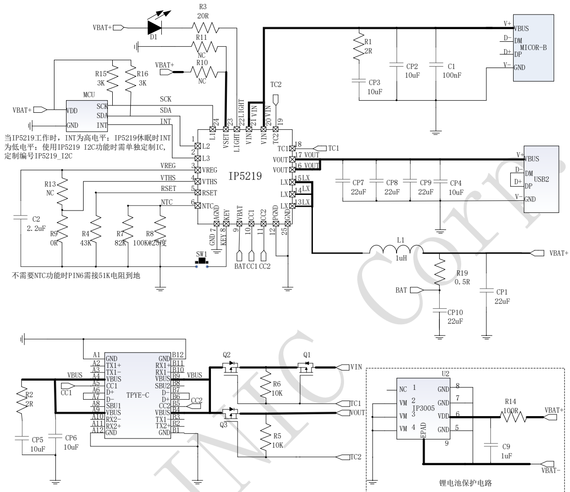
图 7 I2C 典型应用原理图
