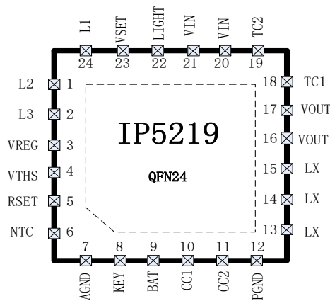
图 2 IP5219 引脚图
