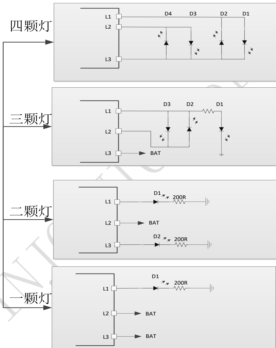
图 4 灯显模式
