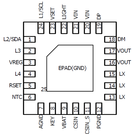
图 2 IP5209U 引脚图
