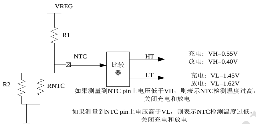
图 5 电池 NTC 比较
