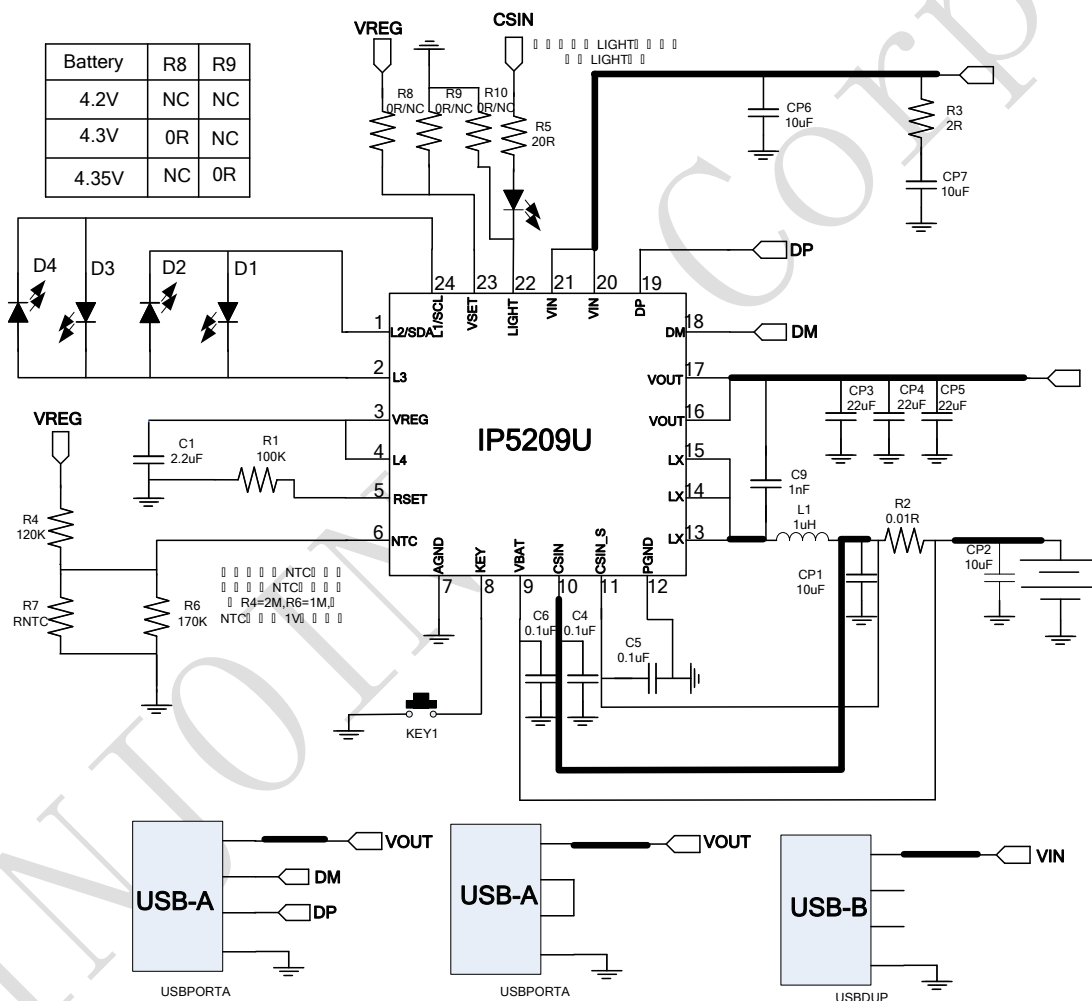
图 6 4LED 电量显示典型应用原理图
