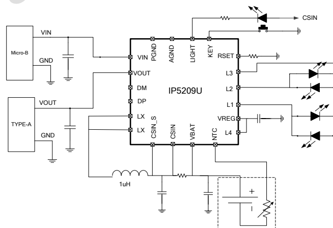
图 1 简化应用原理图(4 LED 指示电量)
