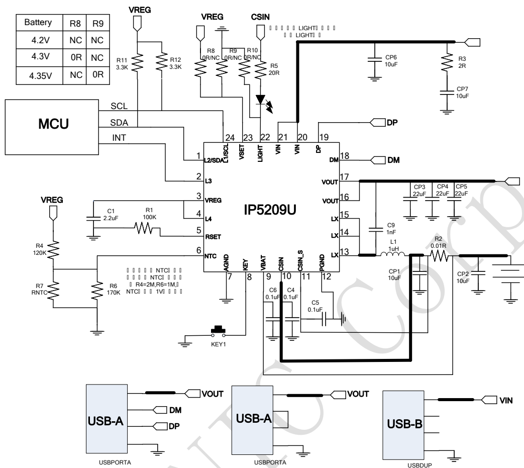
图 7 I2C 应用的典型应用原理图
